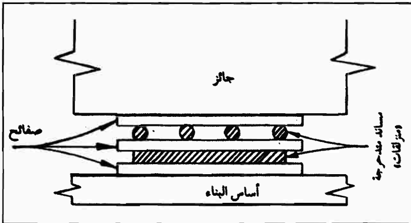
شكل (١٦): أحد طرق تصميم الأساسات لمجابهة الزلازل (٢) .
