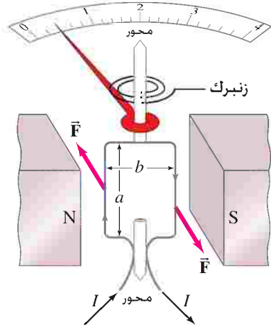
الشكل 20 - 33 جلفانوميتر
