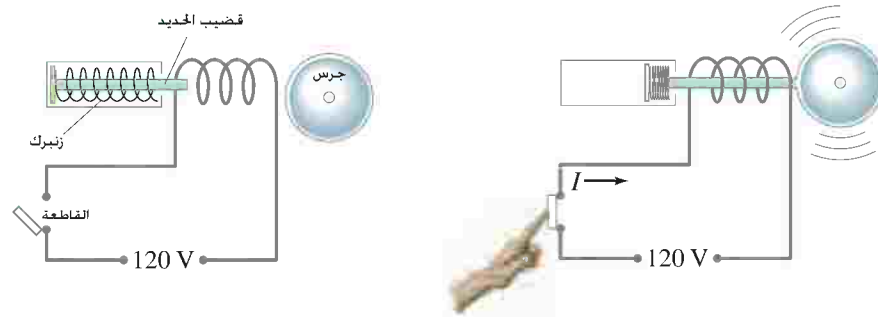
الشكل 20 - 27 الملف الحلزوني المستخدم في جرس الباب.
