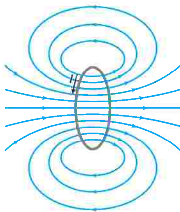
الشكل 20 - 9 خطوط المجال المغناطيسيّ الناتج من حلقة تحمل تياراً كهربائياً.
