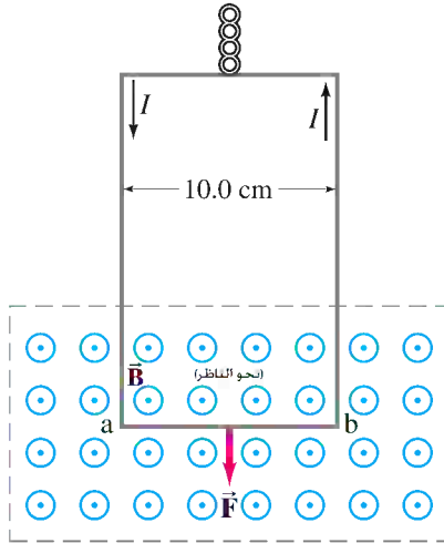
الشكل 20-13 قياس المجال المغناطيسي \vec{B} . المثال 20-2.
