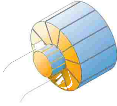
الشكل 20 - 37 محرك كهربائي بعدة لفات
