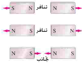
الشكل 20 - 2 الأقطاب المتشابهة
