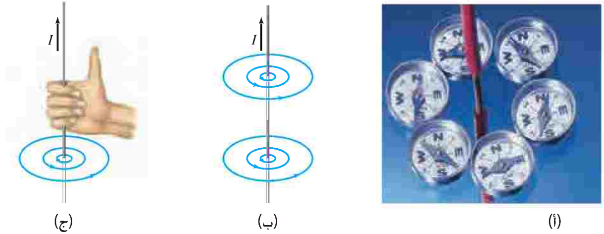
الشكل 20 - 8 (أ) انحراف إبرة البوصلة بالقرب من سلك يحمل تياراً كهربائياً يربنا وجود مجال مغناطيسيّ ويبيّن اتجاهه. (ب) خطوط المجال المغناطيسيّ حول سلك مستقيم يمرّ فيه تيار كهربائيّ. (ج) قاعدة اليد اليمنى لتحديد اتجاه المجال المغناطيسيّ: إذا أشار الإبهام إلى اتجاه التيار الكهربائيّ، فإنّ الأصابع الأخرى تشير إلى اتجاه المجال المغناطيسيّ.
