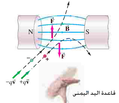
الشكل 20 - 14 القوة المؤثرة في جسيمات مشحونة متحركة في مجال مغناطيسي عمودياً عليه.
