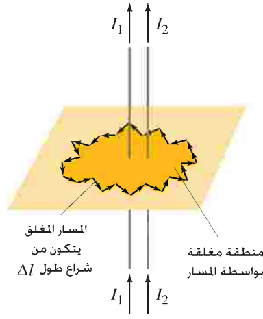
الشكل 20 - 28 مسار اختياري يحوي تيارين كهربائيين للتعامل مع قانون أمبير. قسّم المسار إلى قطع طول كلّ منها \Delta l . التيار الكليّ الذي يحويه المسار المغلق الموضح في الشكل هو I_{\text{encl}} = I_1 + I_2 .
