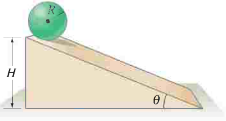
الشكل 24-8: كرة تتدحرج إلى أسفل منحدر لها طاقتين؛ انتقالية ودورانية. (المثال 13-8).
