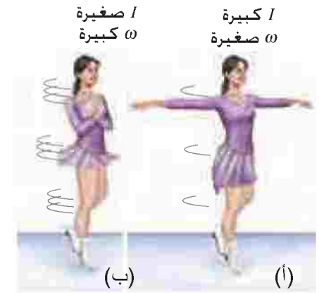
الشكل 8-28: متزلجة تقوم بحركة مغزلية دورانية على الجليد، موضحة حفظ الزخم الزاوي. ففي (أ) I كبيرة ولكن \omega صغيرة؛ وفي (ب) I صغيرة ومن ثم \omega كبيرة.
