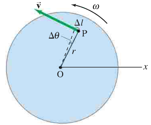
الشكل 8-4 نقطة P على دولاب دائر لها سرعة خطية \vec{v} عند أي لحظة.
