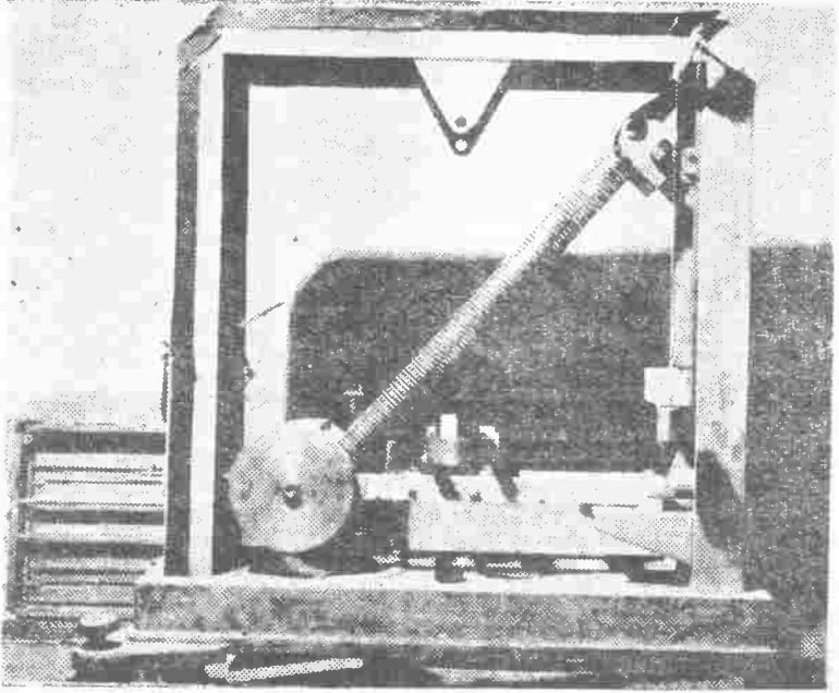
آلة السموتر المستعملة لتسجيل الزلازل الطويلة المدة وهي موجودة بمرصد « لامونث » الجيولوجى التابع لجامعة كاليفورنيا .
