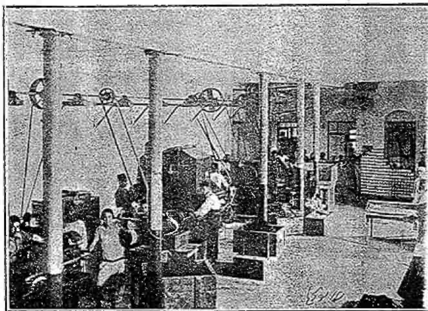
ما كنة لف السجائر . وفرم الدخان واستخراج التيكوتين في معمل حزبون
