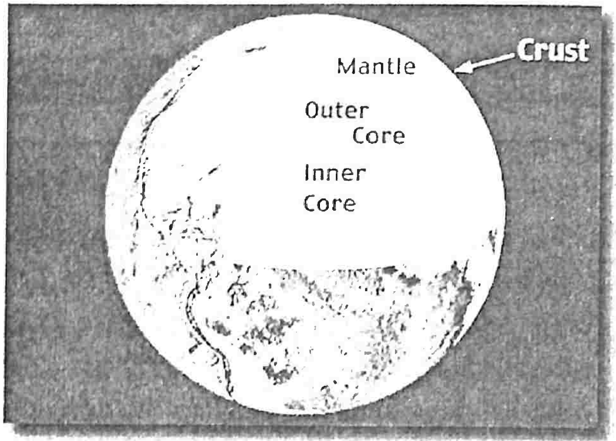
الشكل رقم (١): طبقات الأرض المختلفة من الباطن الداخلى والخارجى وحتى القشرة والسطح يظهر فى باقى الدائرة.
