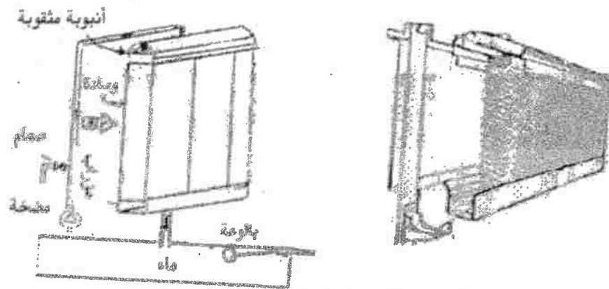
شكل (١٩) التبريد في العناير المفقولة بنظام الوسائد
