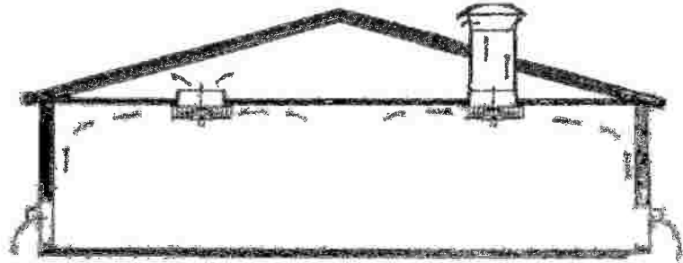
شكل ( ١٤ ) : نظام الضغط الموجب (التهوية في المناير القفولة) مراوح مستطاب
