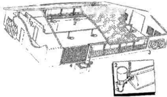
شكل (١٧): التدفئة داخل العنابر باستخدام المولدات
