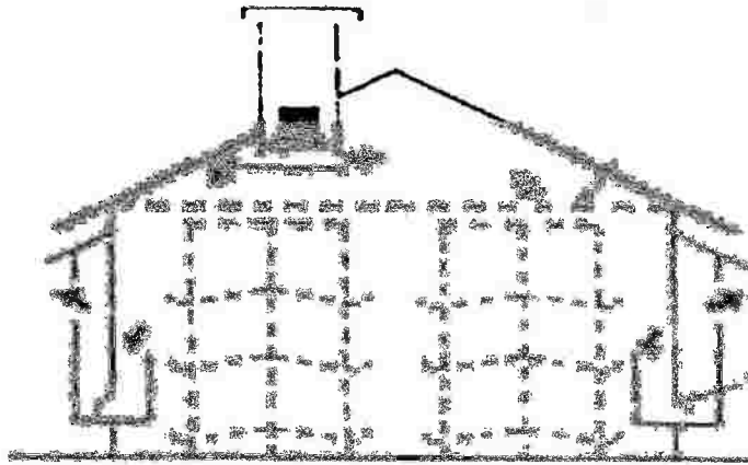
شكل ( ١٥ ) التهوية بنظام الضغط الموجب
