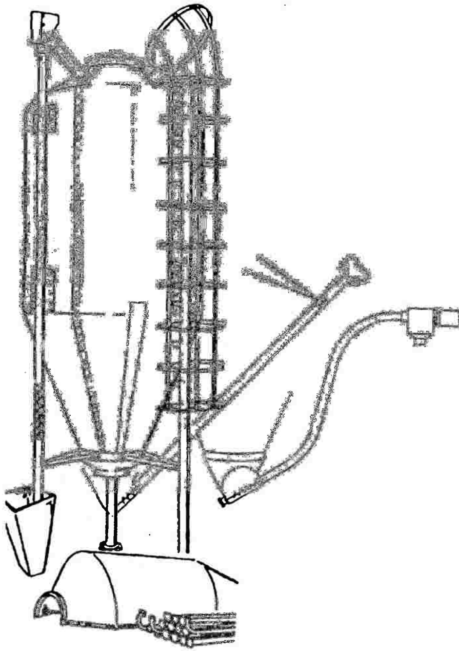
سكر (٢٨) الصومعة لتخزين الملاط لمدة ٧ - ١٠ أيام
