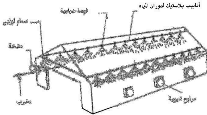
شكل (٢١) : التبريد بنظام الضغط العالي
