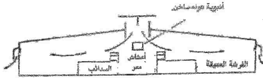
شكل ( ١٣ ) : تيار الهواء العكسي وفتحات السقف للتهوية
