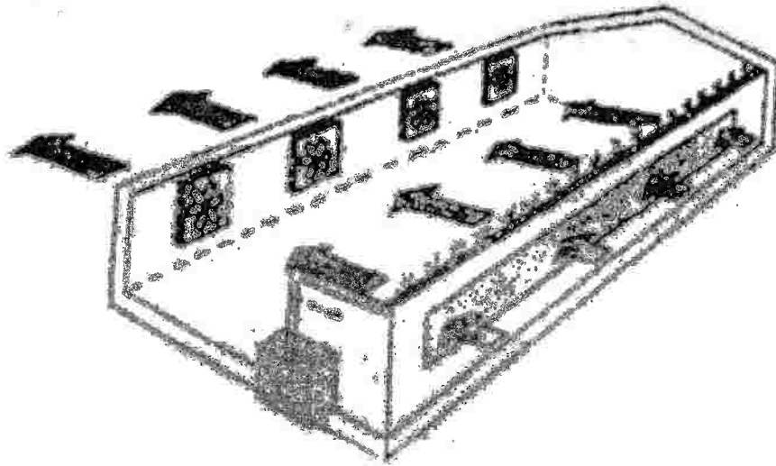
شكل (٢٠) التبريد بنظام الضباب
