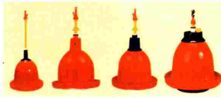
شكل (٢٢) المساقى الأوتوماتيكية (المستديرة المعلقة)
