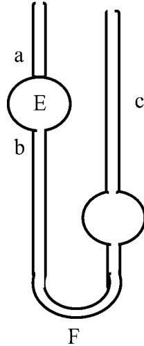
شكل (8) فسكوميتر استفالذ
