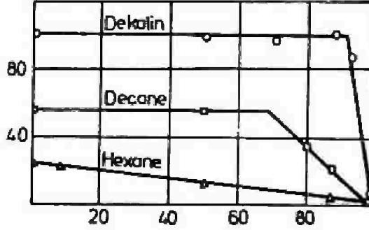
تأثير تركيز الحامل علي العوامل المساعدة من أوكسيد الكروم
