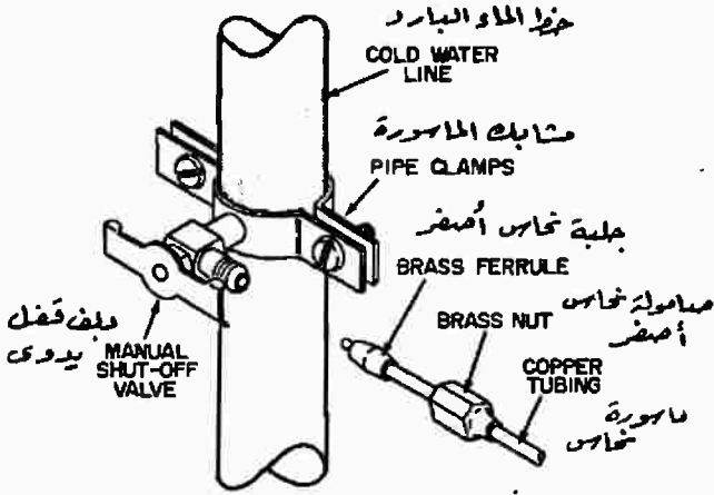
رسم رقم (٦-٢١) - توصيل خط تغذية الماء بالبلف السرج
