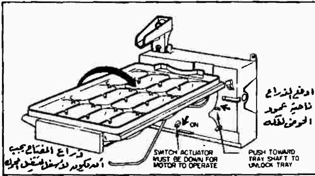
رسم رقم (٦-١٨) - تشغيل جهاز صناعة الثلج يدويا
