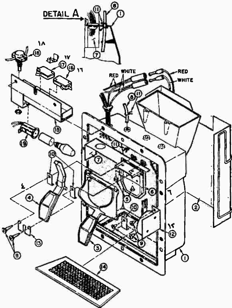
رسم رقم (٦-٢٧) - الأجزاء الخلفية التي تشتمل عليها وحدة توزيع الثلج والماء
