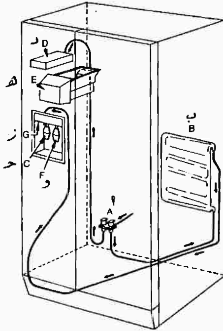
رسم رقم (٦ - ١٩) - مكان أجزاء وحدة توزيع الثلج والماء في كابينه الثلاجة
