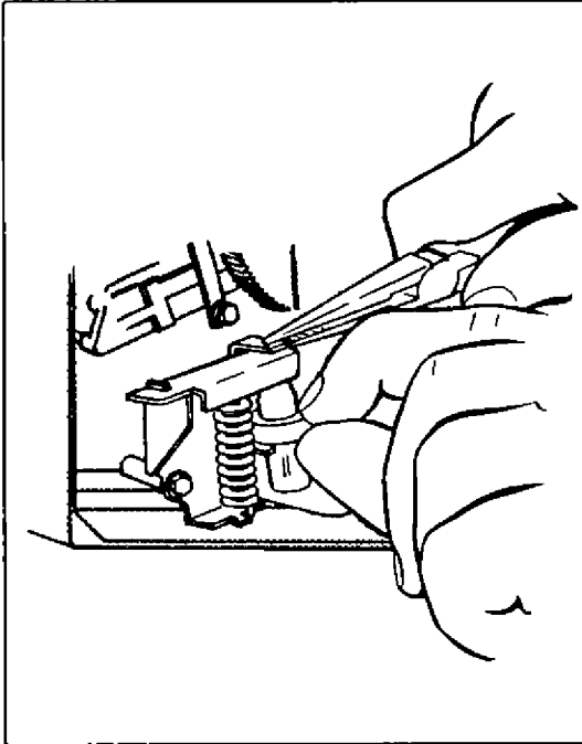
رسم رقم (٦-١٦) - استبدال وحدة الحس الحرارية
