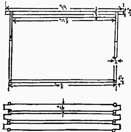
الإطارات من الجانب ومن القمة شكل (١٦)
