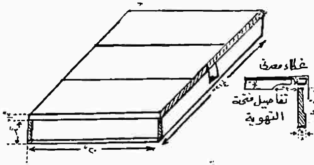
(شكل ٢٠) غطاء خارجي لخلية دادنت المعدلة
