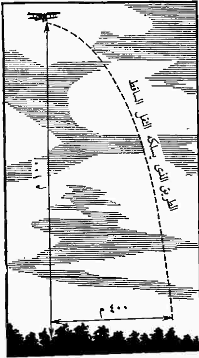
شكل رقم ( ٨ ) إن القل الرمي من الطائرة ، لا يسقط على الأرض بصورة عمودية ، ولكنه يسقط بخط منحن
