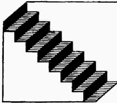
شكل رقم ( ١٣ ) ما الذى يراه القارئ فى هذا الشكل ، هل هو سلم أم تجويف أم شريط منثنى على هيئة أكورديون ؟
