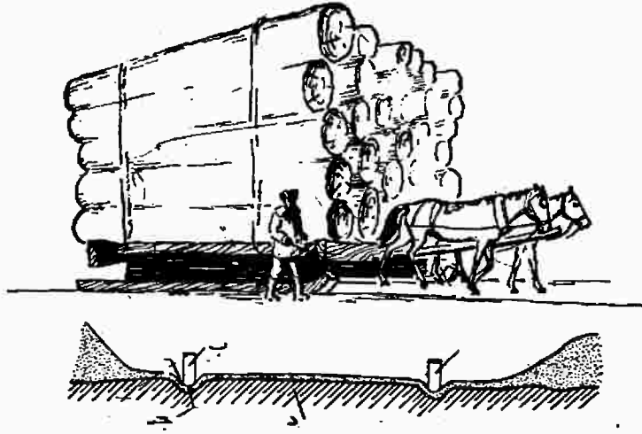
شكل رقم ( ٢ ) الرسم العلوى - زحافة محملة تسير على طريق جليدى : والمخصنان يجران حملاً يبلغ وزنه ٧٠ طناً . الرسم السفلى - الطريق الجليدى : ( ١ ) مسلك الزحافة : ( ب ) المزقة : ( جـ ) جليد مترابط : ( د ) القاعدة الأرضية للطريق .
