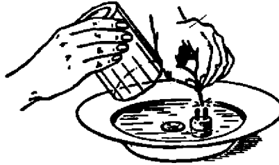
شكل رقم ( ١٠١ ) كيفية التقاط قطعة النقود من الماء بدون تيليل الأصابع
