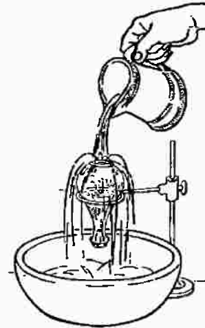
شكل رقم ( ١٠٢ ) إن الماء يغلى فى الفئينة ، عندما نصب الماء البارد عليها
