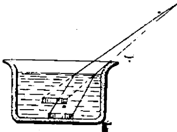
شكل رقم ( ١٢٣ ) السبب الذى يجعل قطعة النقود البيئة في الشكل ( ١٢٢ ) تبدو في موضع أعلى من موضعها الحقيقى
