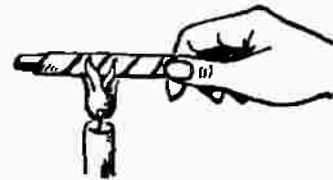
شكل رقم ( ١١٠ ) الورقة التي لا تشتعل
