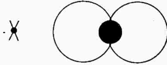
شكل رقم ( ١٢٨ ) الرسم الذى يساعد على اكتشاف البقعة العمياء
