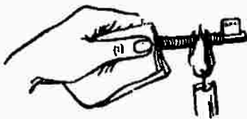
شكل رقم ( ١١١ ) الحيط الذي لا يشتعل
