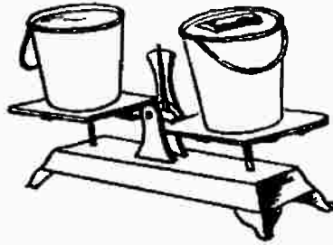
شكل رقم ( ١٠٦ ) إن الدولين هنا مليئان بالماء حتى نهايتهما ، وتطفو على سطح الماء في الدولو الأول قطعة من الخشب . أى الدولين أثقل من الآخر ؟
