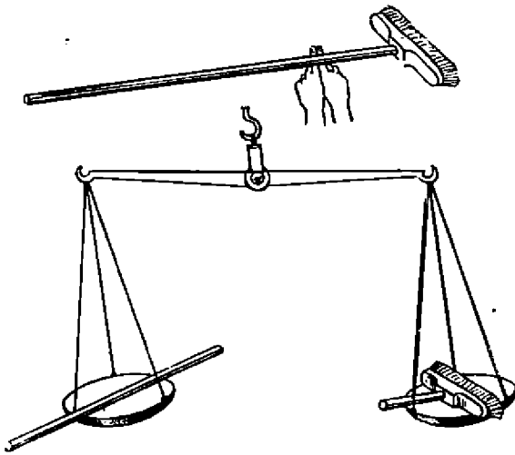
شكل رقم ( ١١٣ ) إجراء نفس التجربة السابقة باستخدام المكسة لماذا لا تتزن كفتا الميزان ؟
