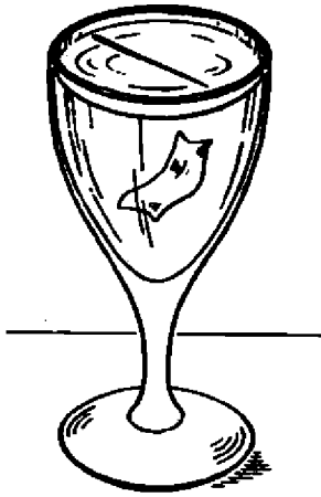
قطعة نقود لا تغوص في الماء
