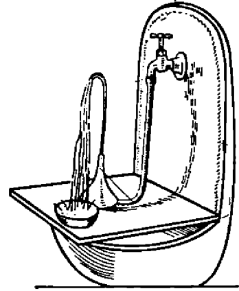
شكل رقم ( ١١٩ ) عاصفة رعدية في الغرفة
