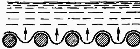
شكل رقم ( ١١٤ ) لماذا لا ينسكب الماء من الغربال المدهون بالبارافين ؟
