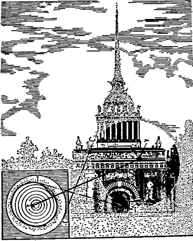
شكل رقم ( ١٢٩ ) عند النظر إلى المبنى بعين واحدة . فإننا لا نرى شيئاً ذلك الجزء الصغير ( حـ ) من مجال الإبصار ، المناظر للقيمة العمياء
