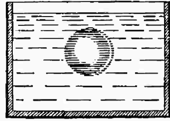
شكل رقم ( ٩٧ ) إن الزيت الموجود في داخل إناء به كحول مخفف ، يتجمع على هيئة قطرة كبيرة ، لا تنفطس في الكحول ولا تطفو على سطحه ( تجربة بلاتو )
