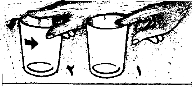
شكل رقم ( ١١٧ ) نفقة من الأكواب
