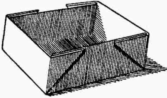
شكل رقم ( ١٠٩ ) صندوق صغير من الورق لعل الماء
