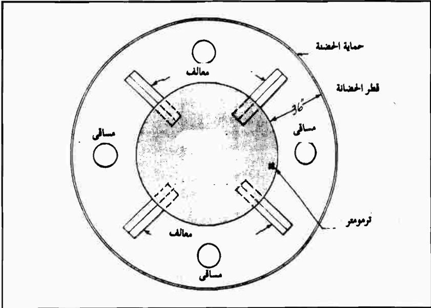
توزيع المعالف والمساقى داخل حاجز الكتاكيت أسفل الدفايات
