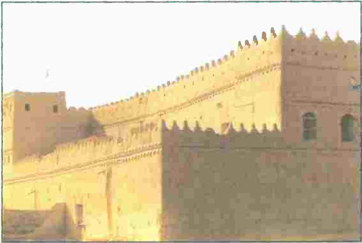
صورة (١٧): جانب من منزل كبير تظهر فيه دقة الطراز المعماري ١- شرف ٢- حداير ٣- حقاف
