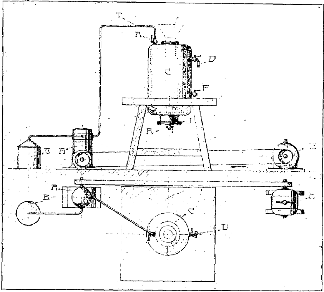
الشكل السادس عشر — صورة الجهاز الذي استعمل في اختبار تبخير بذرة القطن بغاز حمض السياندريك في الفراغ
