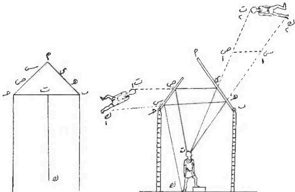
( ٤٧ ) وضع مرآتين مستويتين تظهران انعكاساً مزدوجاً طائرًا في الهواء ( جهاز مرآوي ) ، بحسب القضية ١٥ من كتاب ايون السكندري في د الحيل .
