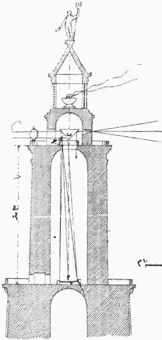
(٣٤) منارة الاسكندرية تليسكوب و نيوتوني . . اعادة تركيب وتصميم تيرش ، ١٩٠٩ (أ) مرآة مقعرة . (ب) مرآة مخروطية مائلة بزاوية ٤٥ درجة . (ج) مشاهد واقف على المنصة العليا .
