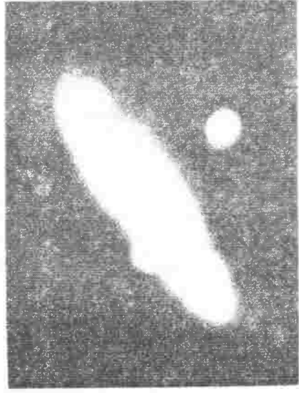
مجرة المرأة المسلسلة (M 31)
