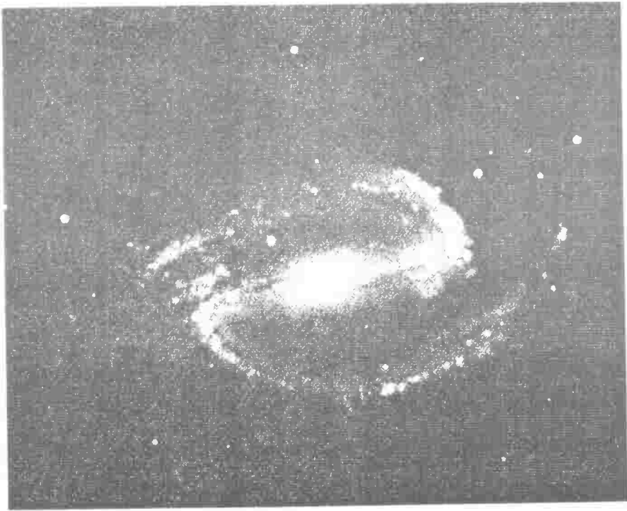
المجرة الحلزونية ذات القضيب (NGC. 1300)
