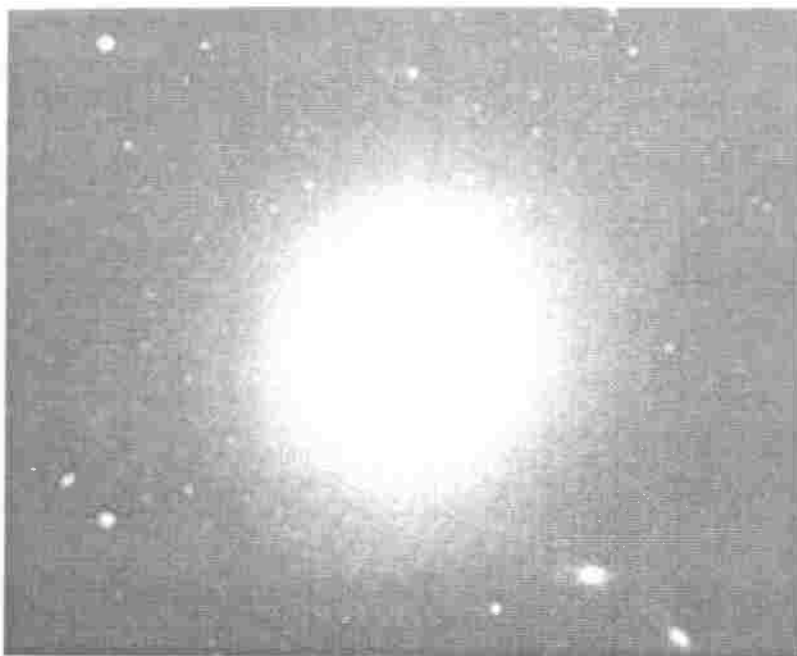
المجرة الإهليجية M 87 التي تقع في قلب حشد العذراء، وهي مثال آخر على هذا النوع من المجرات، وشكلها أقرب للكرة.
