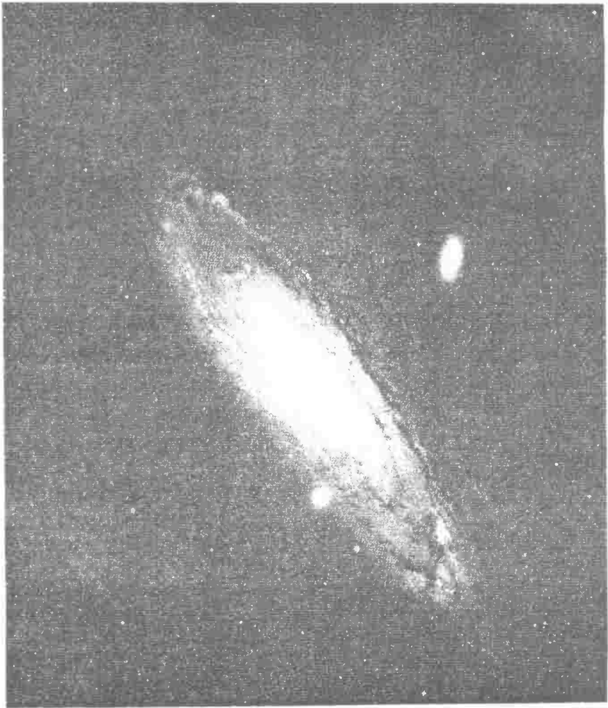
المجرة الحلزونية في كوكبة المراء المسلسلة . (M31)
