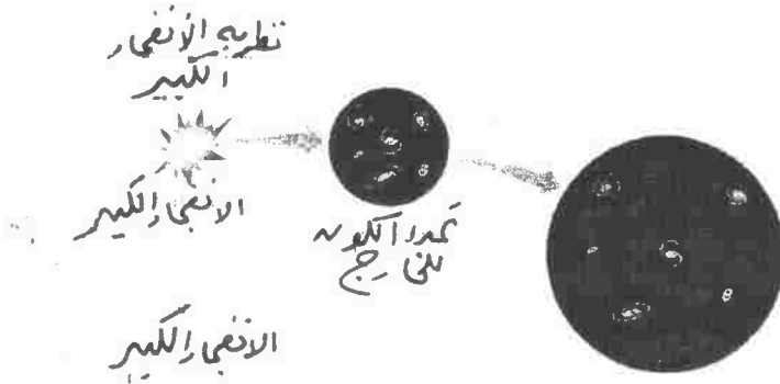
رسماً تخطيطياً للانفجار الأعظم وتوسع الكون
