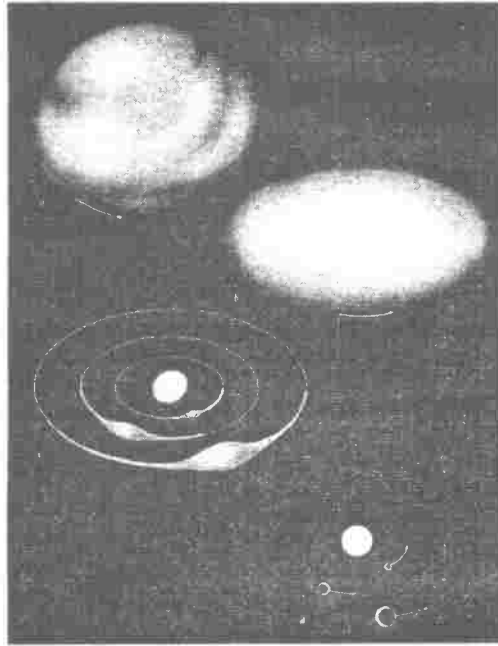
السديم الشمسى
