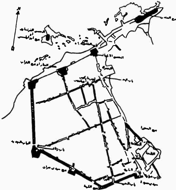
شكل (١٦) أسوار وحصون وأبواب طرابلس سنة ٩١١
