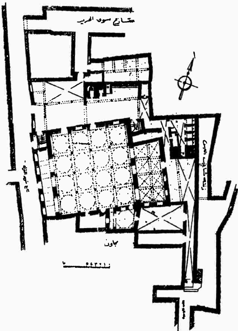
شكل (٥) مسقط أفقي لجامع شاذلي العين (١١١٠هـ/١٦٩٩/٩٨) (عن القسم الهندسي بمصلحة الآثار / طرابلس)
