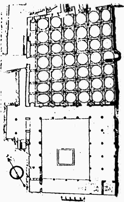
شكل (٣) مسقط أفقي لجامع للناقة . (عمل الباحث)
