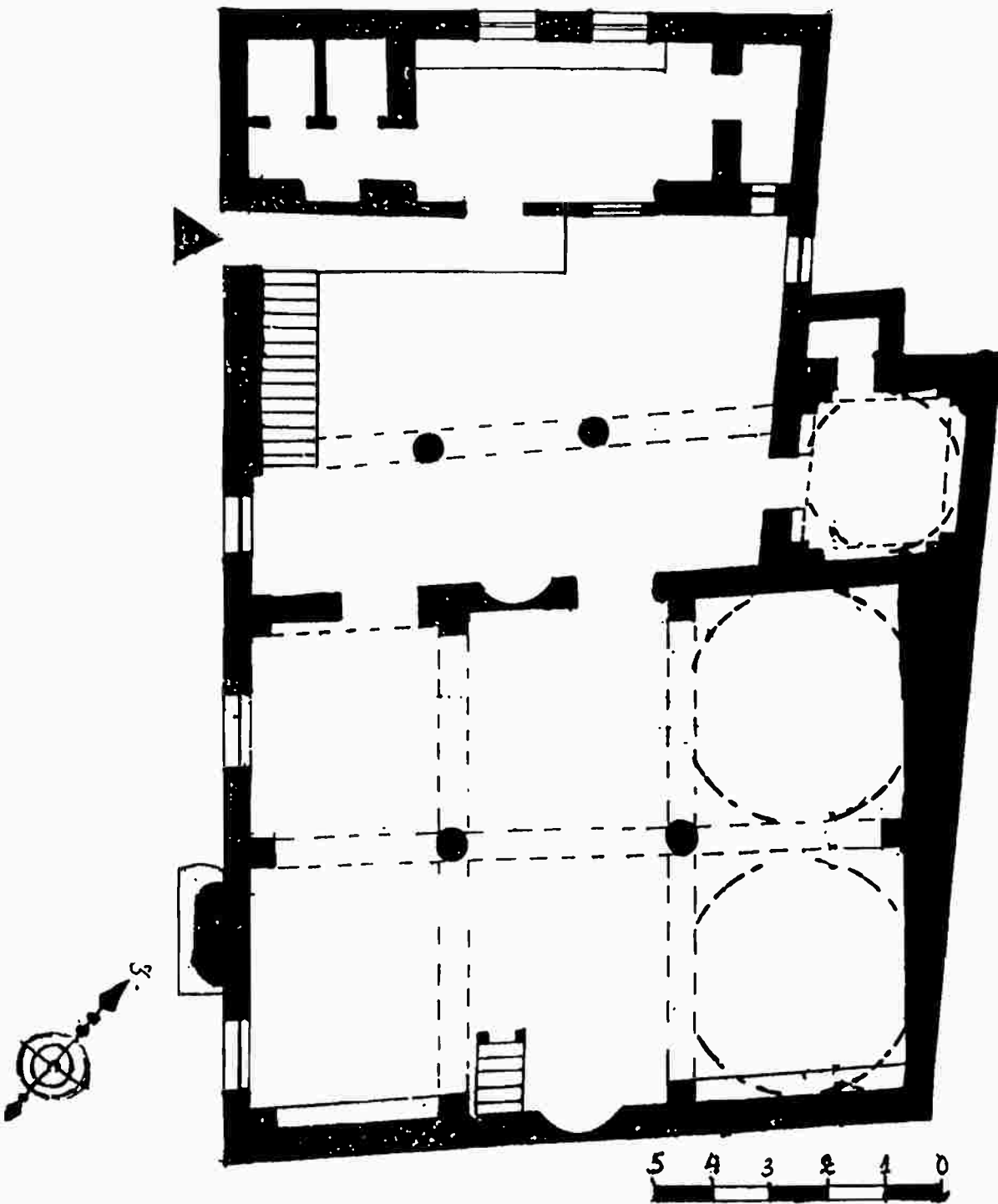
شكل (١١) مسقط أفقي لمسجد بن مقول (النصف الثاني من القرن ١٠هـ / ١٦م) (عمل الباحثة)
