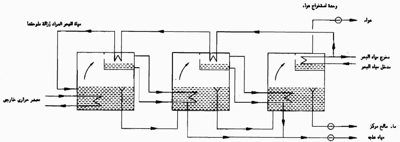
شكل (٢.٢) : وحدة إغذاب المياه ذات المراحل المتعددة
