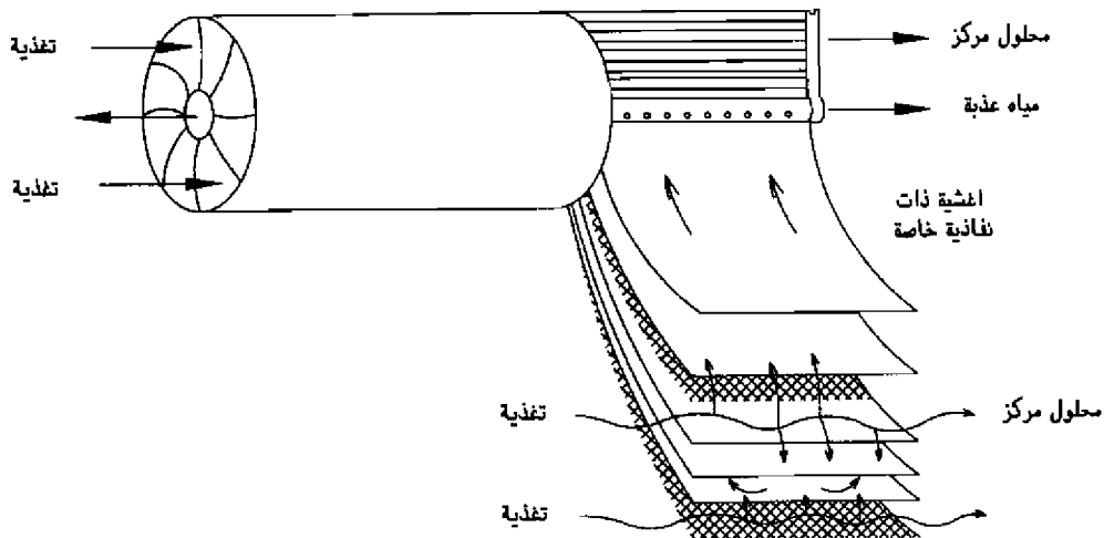
شكل (١٠.٢) ، رسم تخطيطي لنموذج غشاء من النوع المجوف
