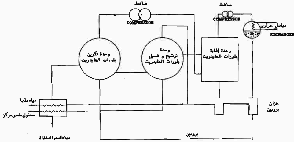
شكل (٢-٨) : تحلية المياه باستخدام الهيدريت
