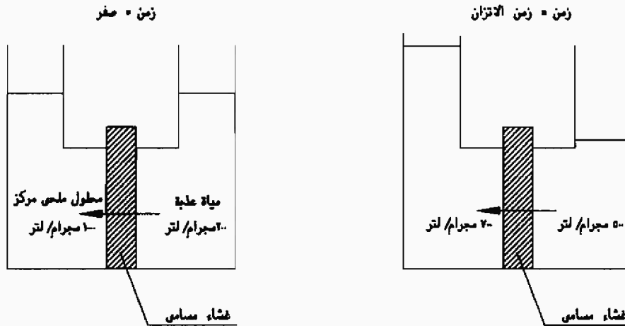
شكل (٨-٣) : التناضح الأسموزي في حالة اتزان
