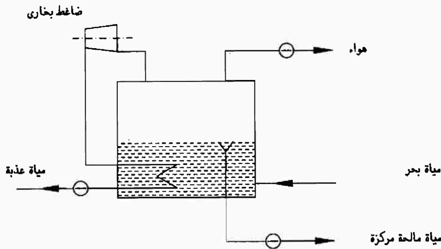
شكل (٦.٣) : وحدة تحليلية مياه بضغط البخار
