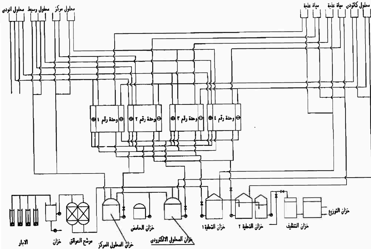
شكل (٣.٤) : محطة إعذاب مياه بالديليزة الكهربائية
