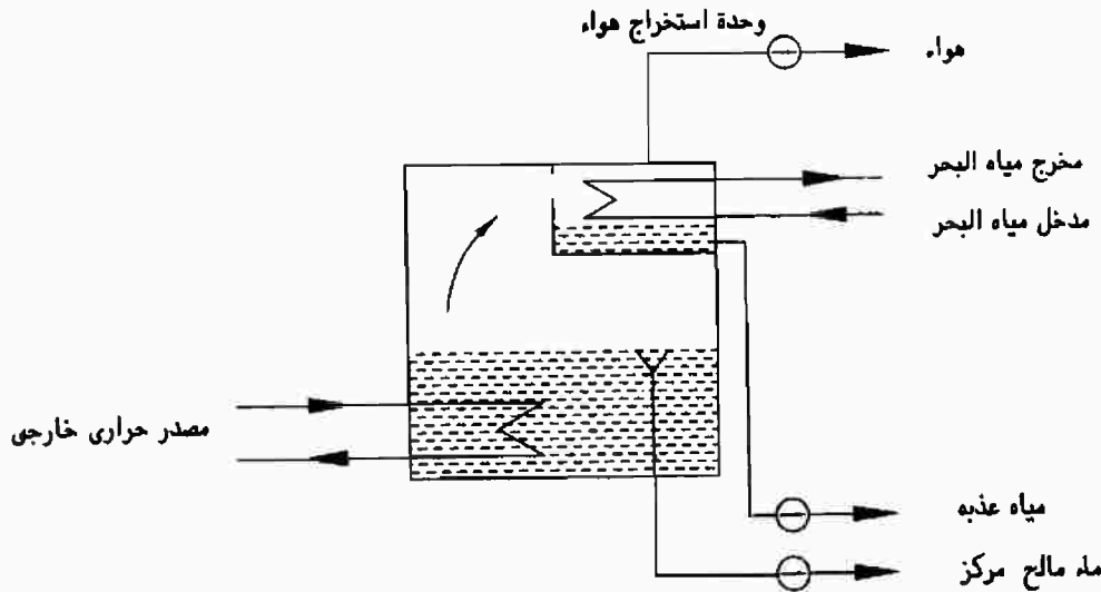
شكل (١.٢) ، وحدة إغذاب المياه ذات المرحلة الواحدة
