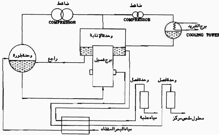
شكل (١-٨) : تحلية المياه بالتجميد
