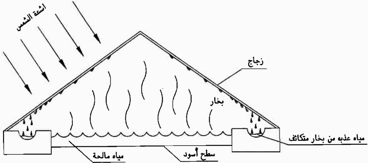
شكل (٧-٢) : مقطر شمسى بسيط للمياه
