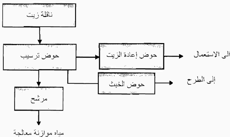
شكل (٧-١٣): مخطط لمعالجة مياه الاتزان للنقلات .
