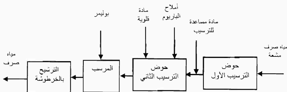
شكل (٤-٦): مخطط يوضح المعالجة الفيزيائية الكيميائية للملوثات إشعاعية.
