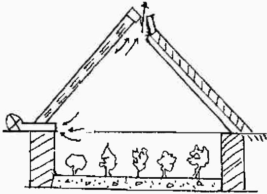
شكل (٩/٤) صوبة صيفية
