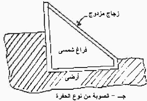
شكل (٩/١) مخطط لمعظم الصوبات الشمسية
