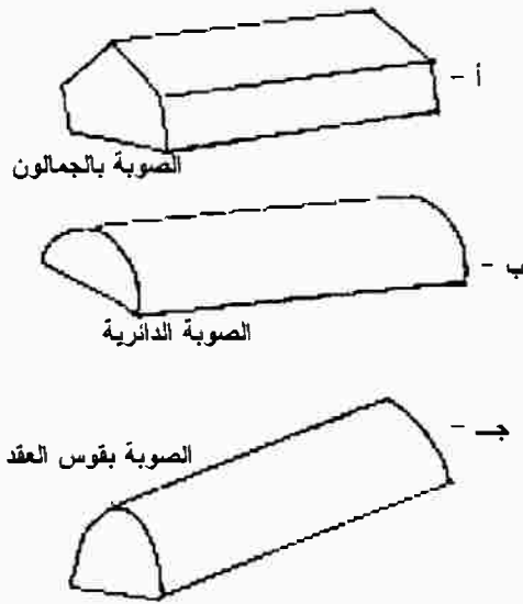
شكل (٩/٢) بعض الأشكال العادية للصوبة
