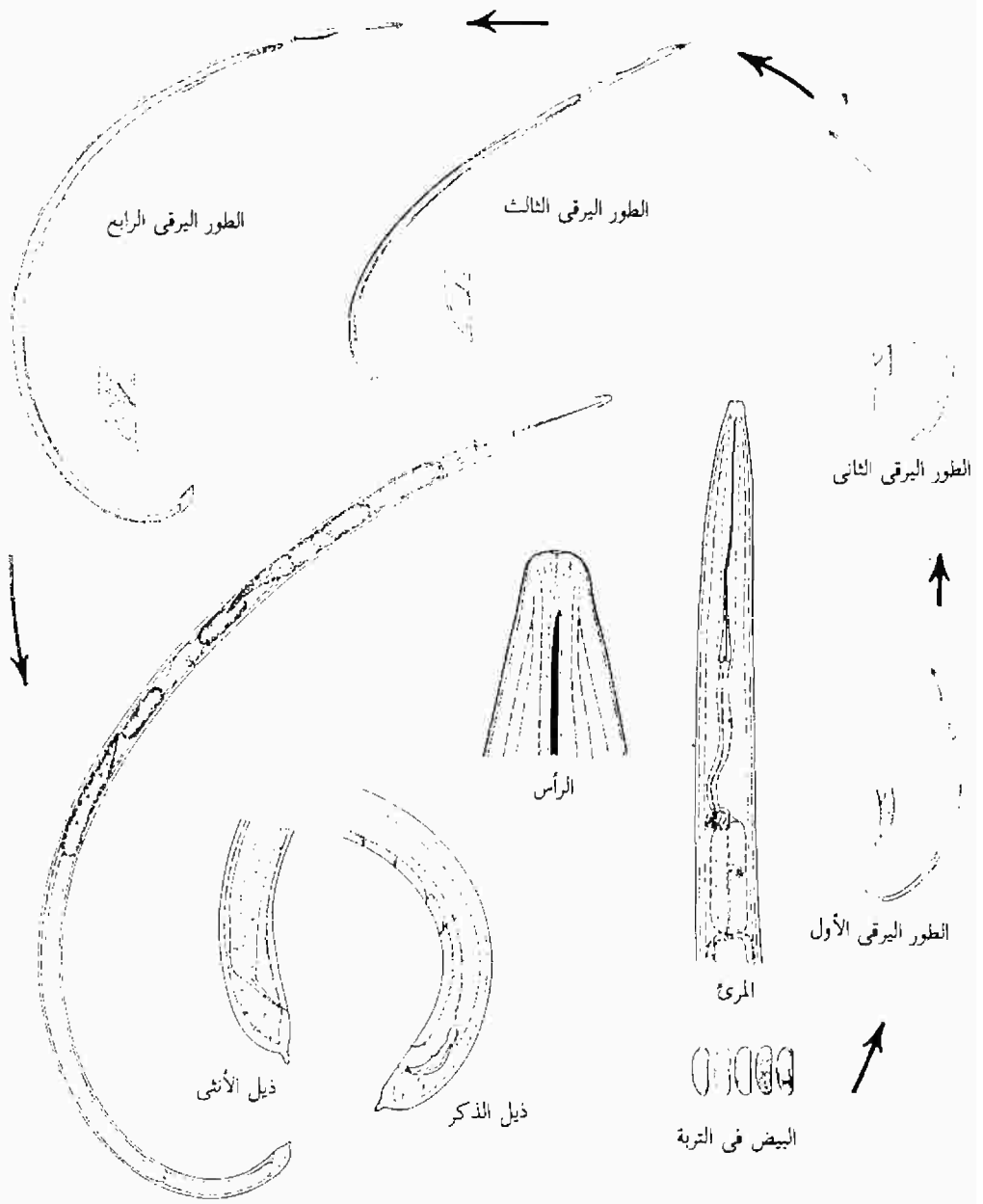
شكل رقم (٢٩) دورة حياة الـنيماتودا الخنجرية
