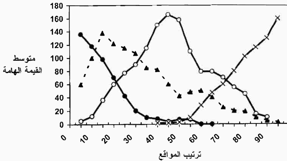
شكل (٧٢). البيانات الأصلية ( أ ) والمنحنيات الملساء (ب) لأربعة أنواع من الأشجار فى الغابات المرتفعة شمال ويسكونسون على مدى تدرج تعاقبى. •: البلوط الأسمر △: البلوط الأبيض، ○: البلوط الأحمر، ×: اسفندان السكر.
