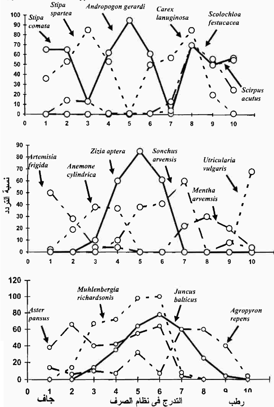
شكل (٧١). توزيع ١٦ نوع نباتي على طول تدرج نظام الصرف فى مقاطعة نيلسون (شمال داكوتا).
