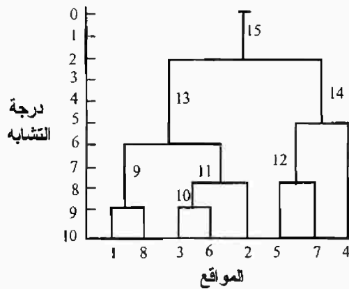
شكل (٦٧). رسم متفرع مبنى على محتوى معلومات المجموعات
