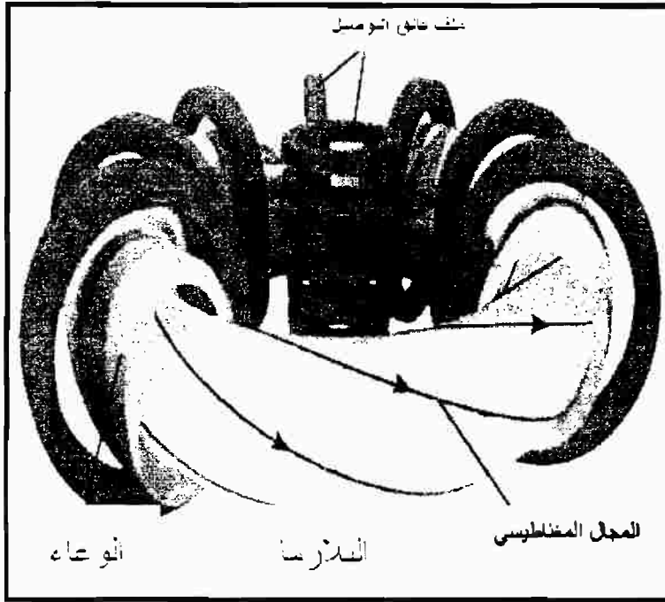
شكل (١٩): المبدأ الذي يعمل بموجبة مفاعل الأيتير.
