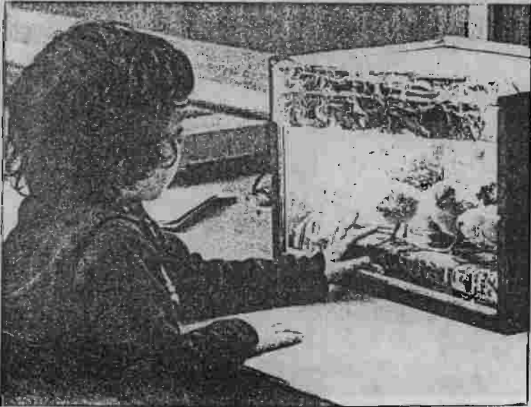
تتبع دورة الحياة والتغذية والمعيشة على الطبيعة
