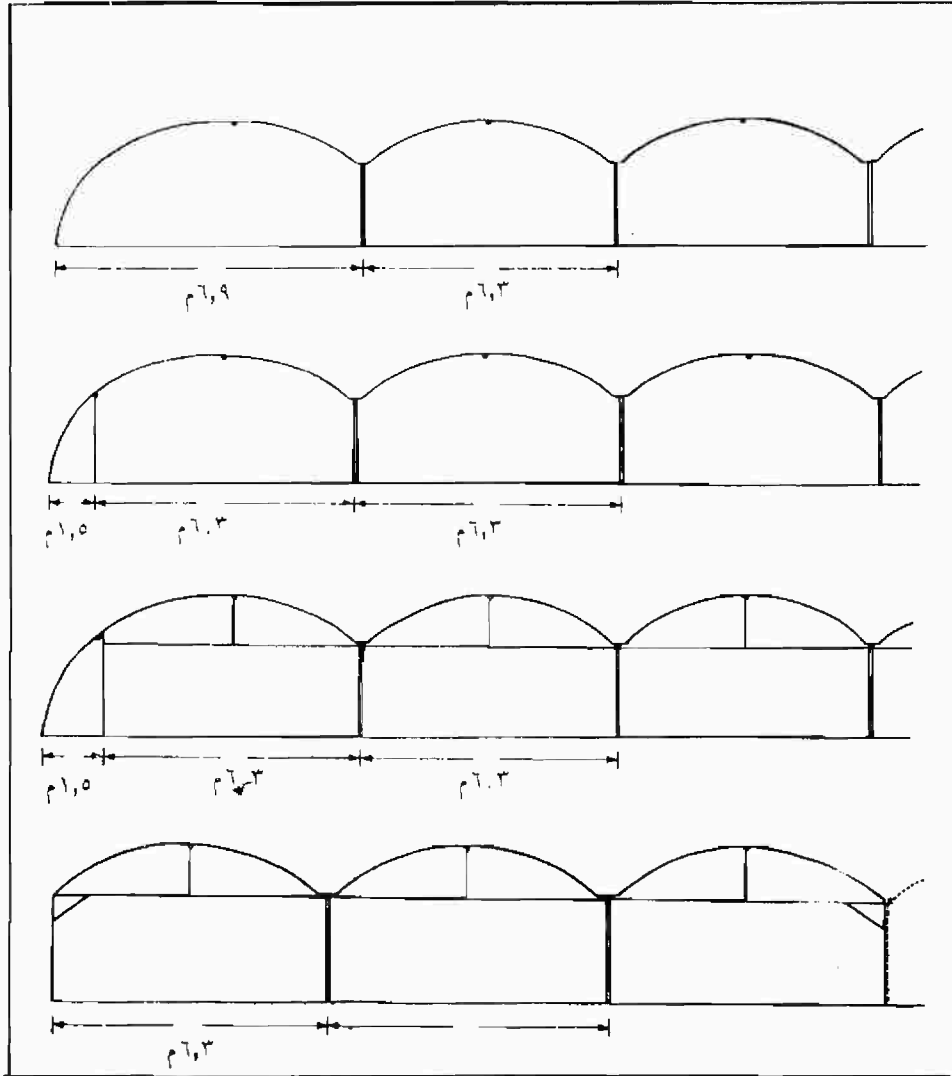
شكل ( ٢ - ٤ ) : مقاطع فى تصميمات مختلفة لمجمعات من البيوت على شكل الخطوط والقنوات تكون من وحدات ذات أسقف منحنية تصلح للغطية بالبلاستيك أو بالفيرجلاس .
