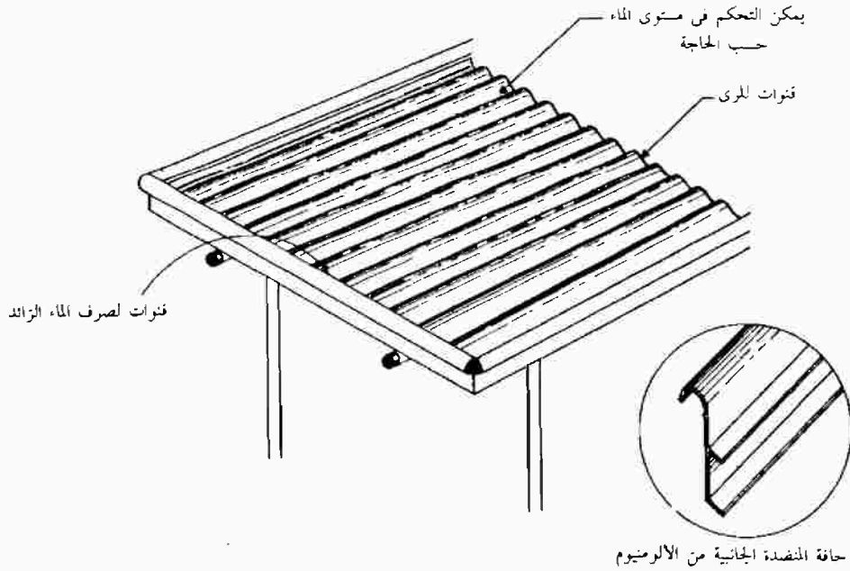
شكل (٢ - ١٤) : رسم تخطيطي لأحد أنواع مناضد الزراعة .
