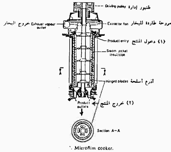
شكل ( ٩ - ٦ ) وحدة طبخ للسكر بنظام الـ Micro Film
