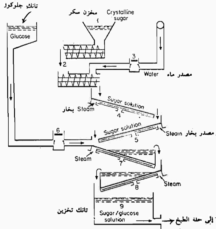
شكل (٩-١) وحدة إذابة مستمرة للسكريات
