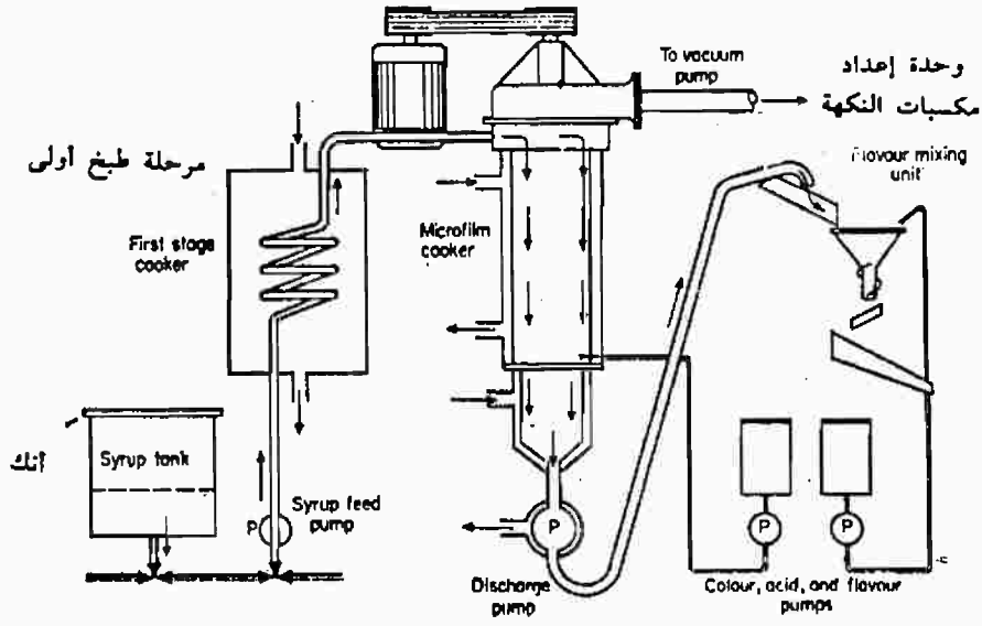
شكل (٤-٩) وحدة إنتاج للحلويات بالنظام المستمر
