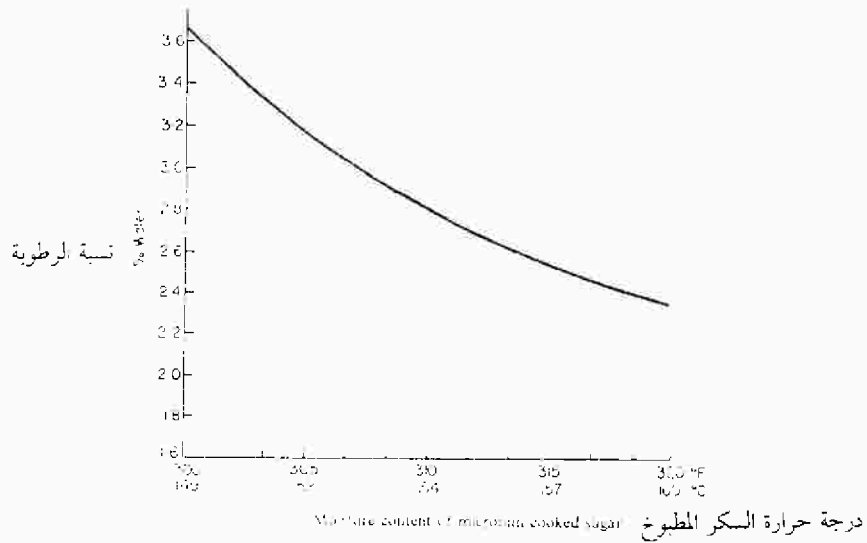
شكل ( ٩ - ٧ ) متابعة للرطوبة أثناء الطبخ للسكر
