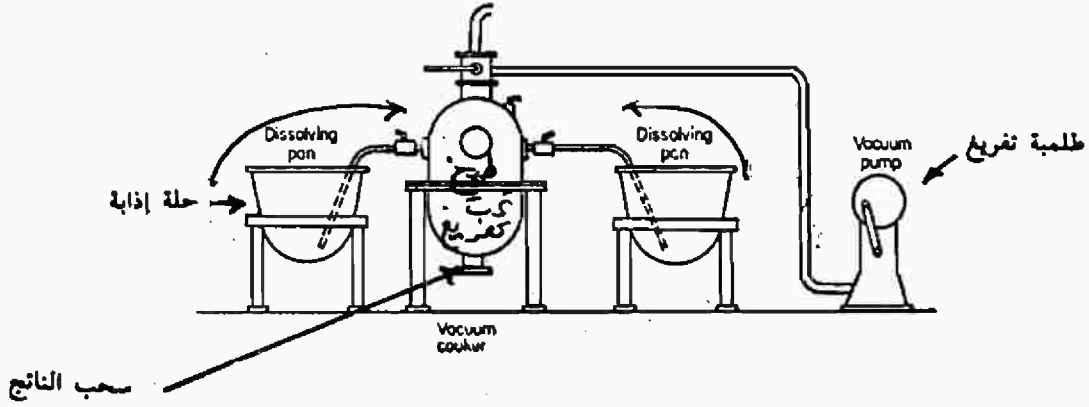
شكل (٩-٣) وحدة طبخ للسكر تحت تفريغ (نظام قديم)
