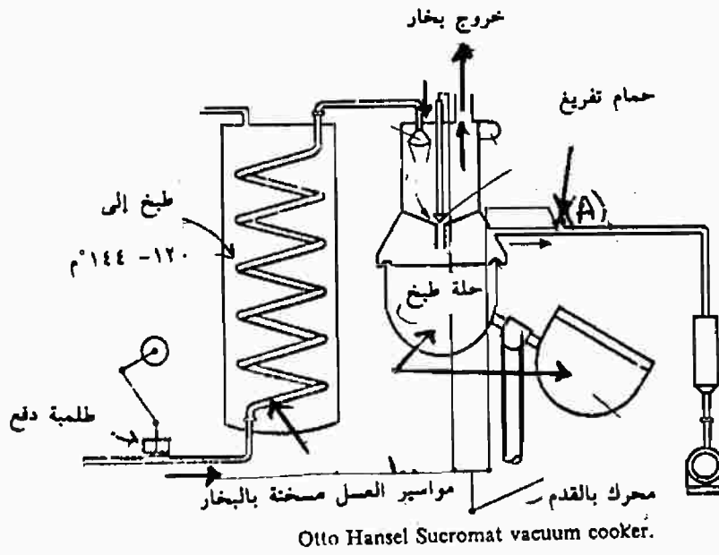
شكل (٥-٩) نموذج لتجهيزات حلة طبخ تحت تفريغ
