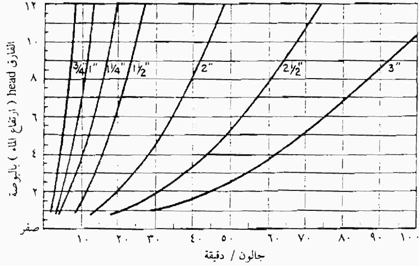
معدل التصريف من سيفونات صغيرة ( قطر السيفون بالبوصة )
