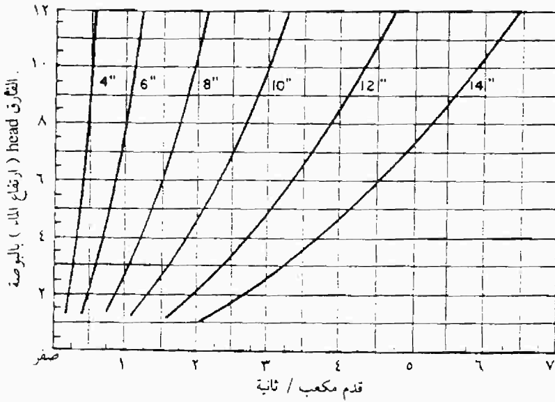
معدل التصرف من أنابيب كبيرة ( قطر الأنابيب بالبوصة )
