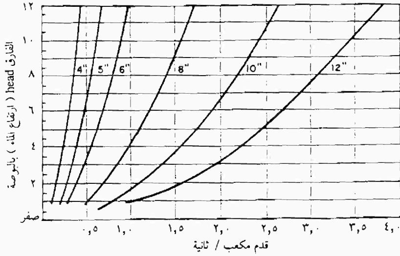
معدل التصريف من سيفونات كبيرة ( قطر السيفون بالبوصة )
