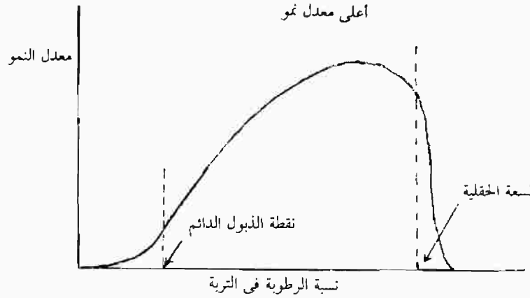
شكل ( ٦ - ٣ ) : تأثير الرطوبة الأرضيّة على معدل النمو النباتي (عن Israelsen & Hansen ١٩٦٢) .
