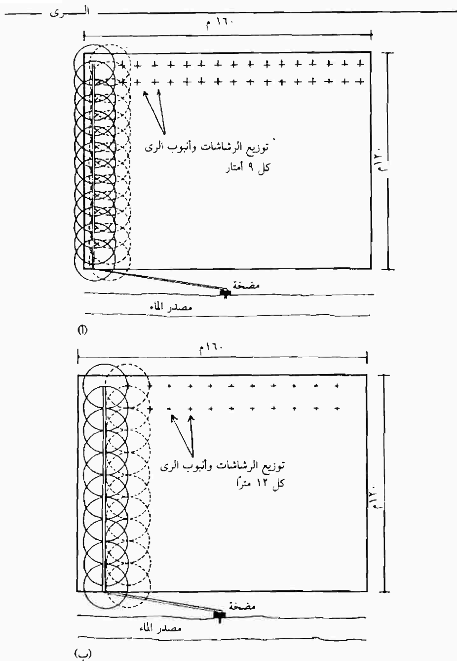
شكل (٦ - ١٤) : التصميمات الممكنة لشبكة ري لحقل تبلغ أبعاده ١٦٠ \times ١٢٠ م تحت الظروف الموضحة في المتن.
