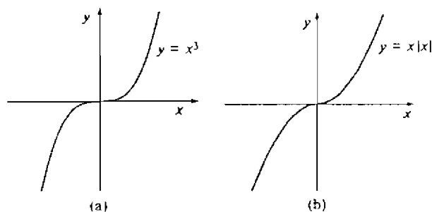
شكل (٦-٣): يبين منحنيات الدالتين y = x|x| ، y = x^3
