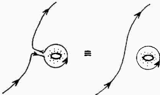
شكل (٧-٢) : يوضح الشكل كيف أنه بالنسبة للمسارات المتشابهة (homologous) تلغى بعض الأجزاء أجزاء أخرى وإن كان ينتج عن ذلك بعض الانشوطات (loops) المنفصلة بعضها عن البعض.
