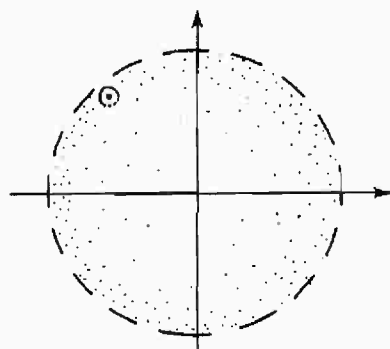
شكل (٤ - ٧) : القرص الوحدة المفتوح - |x| < 1 أما القرص المغلق فى معنى |x| \leq 1 لأنه يتضمن نقاط المحيط.
