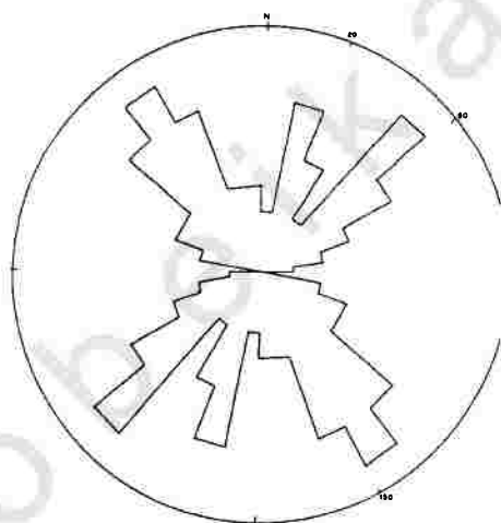
شكل رقم (٤) شكل بياني للتصدعات الطولية العرضية من لاندسات (١)
