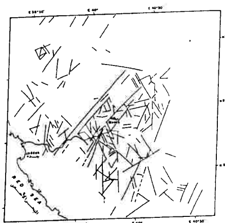
شكل رقم (٣) خريطة تركيبية للشقوق والتصدعات لمنطقة مكة المكرمة (القمر الصناعي لاندسات (١))
