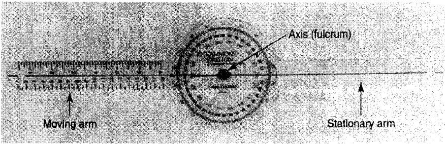
الأشكال المختلفة للجينوميتر
