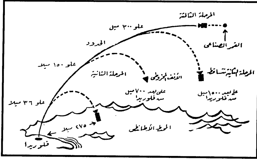
مسار كل مرحلة من مراحل صاروخ الفانجارو ومواقع سقوطها
