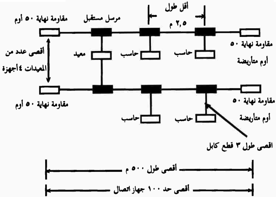
(شكل ٨-٢) قواعد توصيل إيثرنت 10 BASE5
