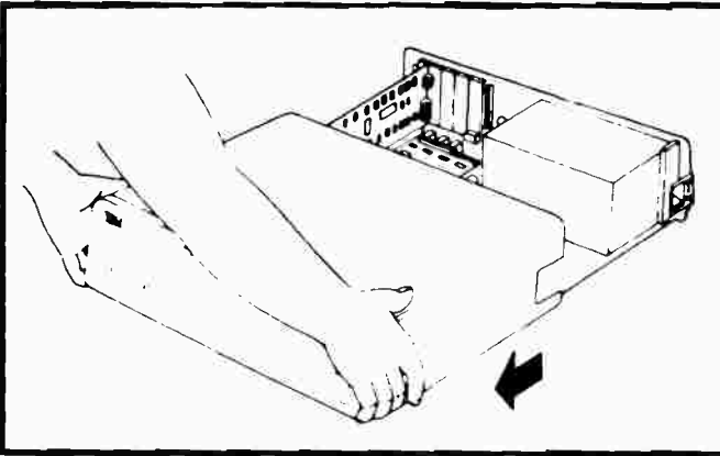
سحب غطاء صندوق النظام
