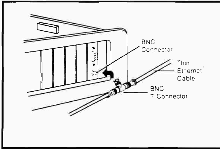
توصيلات الكابل الرفيع فى الشبكة
