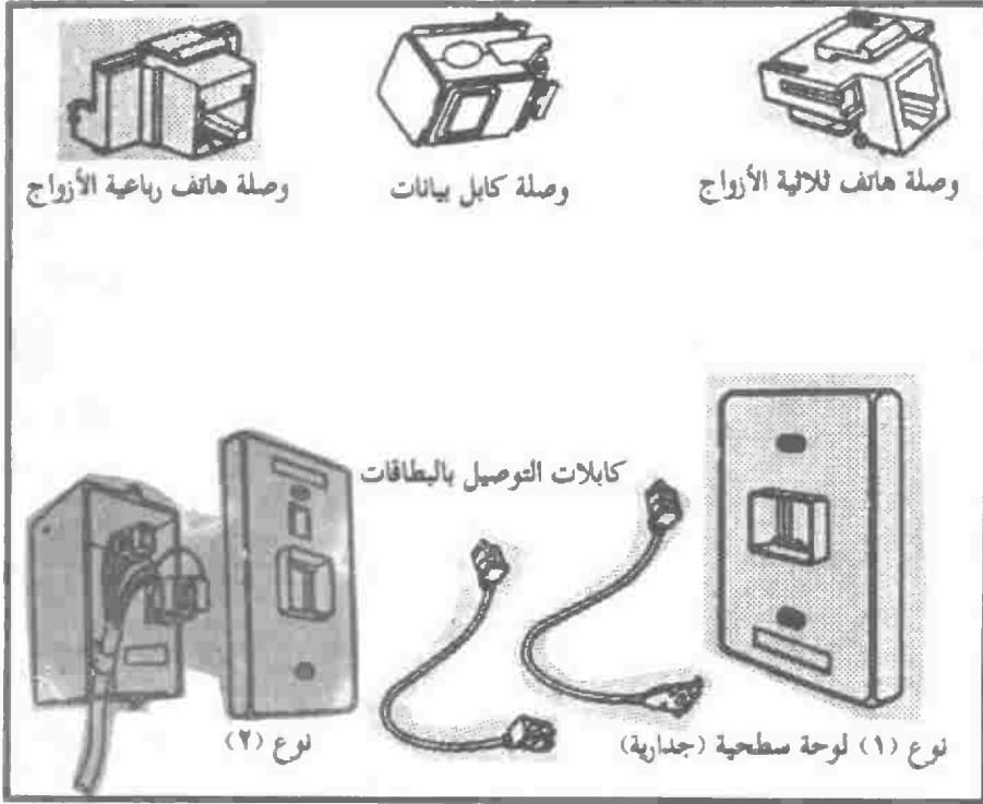
ملحقات توصيل شبكة توكن رنج شكل (٨-٤)
