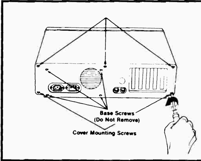
فك مسامير تثبيت غطاء صندوق النظام
