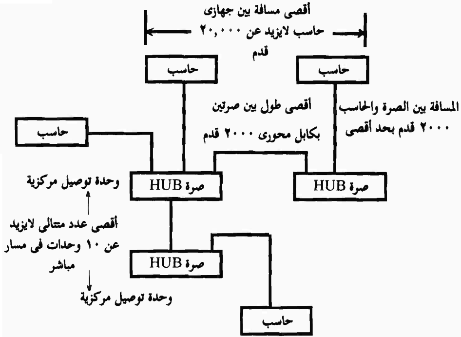
قواعد توصيل شبكة آركنت بكابل محوري (شكل ٨-٥)
