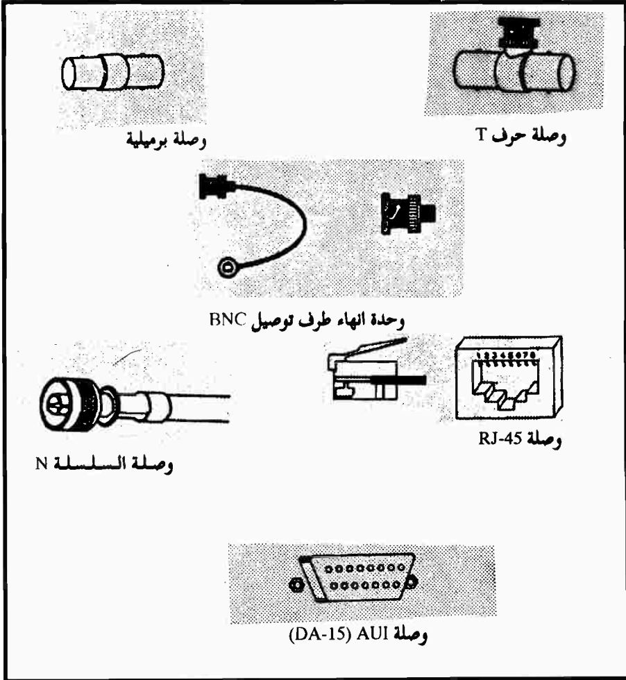
شكل (٨-١) ملحقات توصيل كابلات الايثرنت
