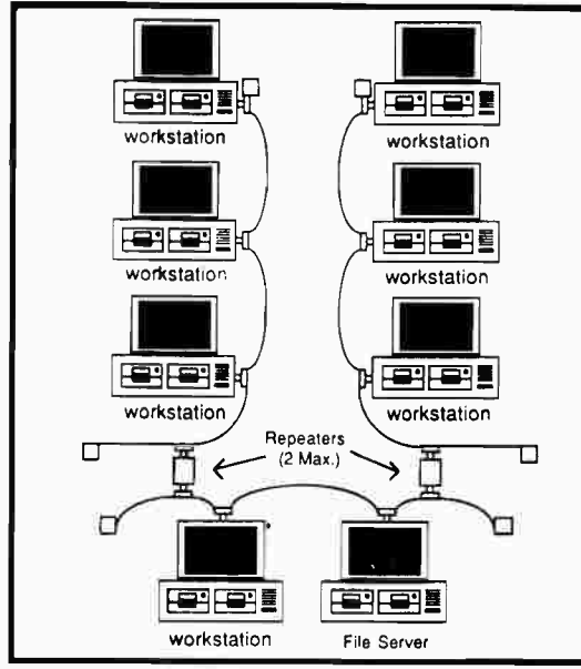
التوصيل باستخدام المعيدات فى شبكة إيثرنت
