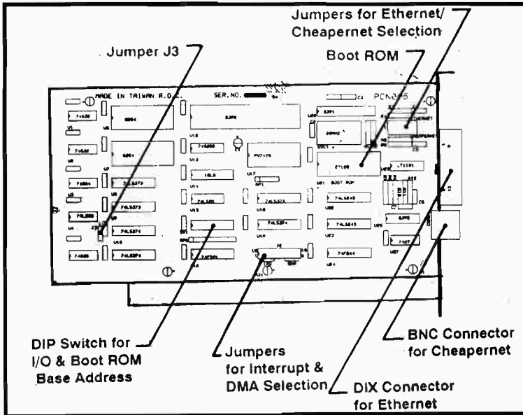
مخطط وظيفى لبطاقة الشبكة
