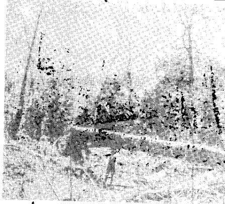
(زلزال نيومدريد في ١٨١١ يفتتق الأشجار)
