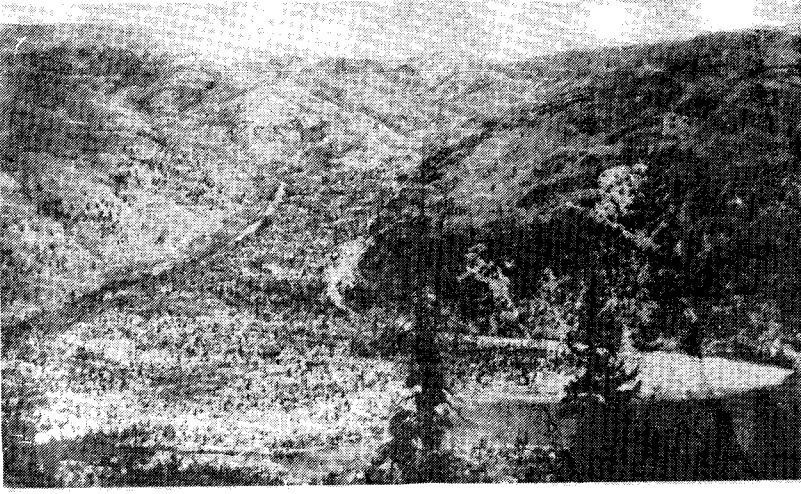
(انتشار فيضاني للطمي فى كلورادو)
