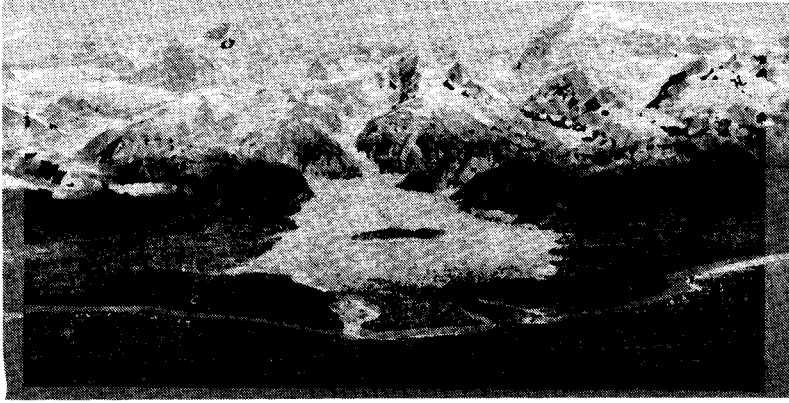
(انزلاق أرضي من خليج ليتويا - آلاسكا في ٢٩ أغسطس ١٩٥٨)
