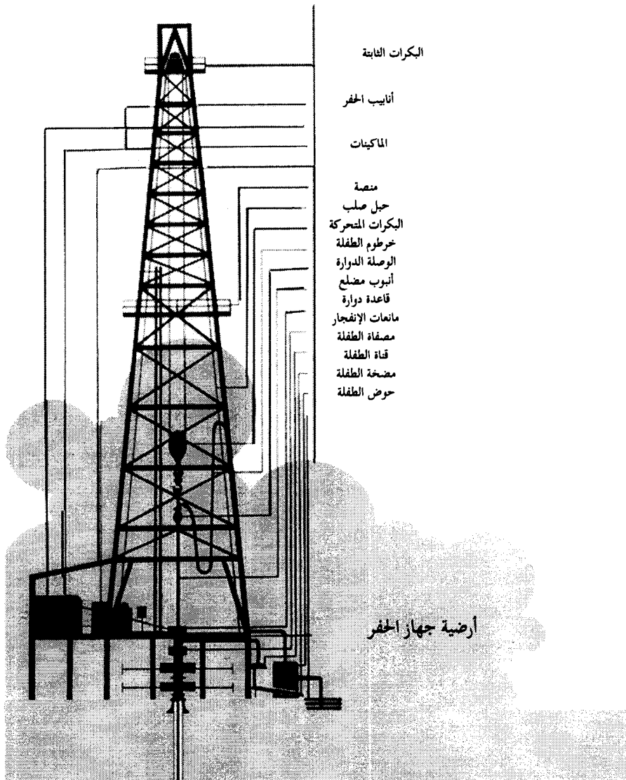
جهاز الحفر الدوار المستخدم في حفر الآبار العميقة مبنيًا عليه الأجزاء المختلفة
