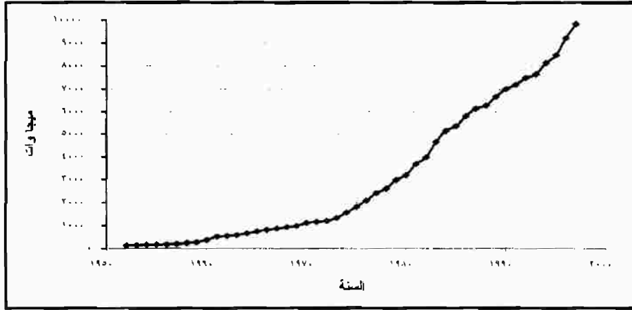
شكل (٢-٢): تطور الحمل الأقصى في الفترة ١٩٩٧-١٩٥٢
