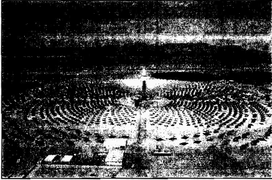
شكل (٢-٦): منظومة البرج المركزي
