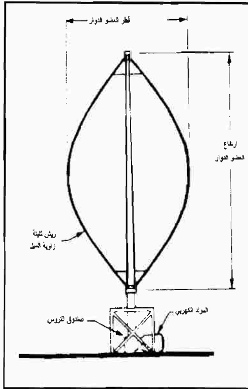
(ب) التوربينات الرأسية
