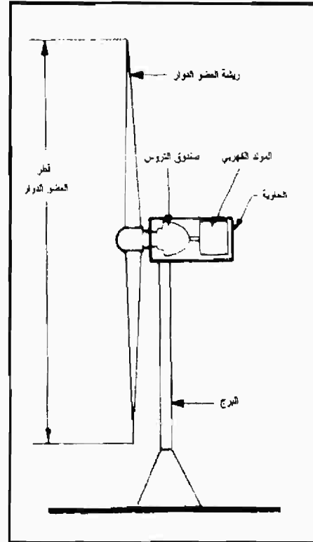
(أ) التوربينات الأفقية
