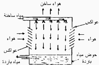
شكل (٩/٥) حوض الرش الهوائي
