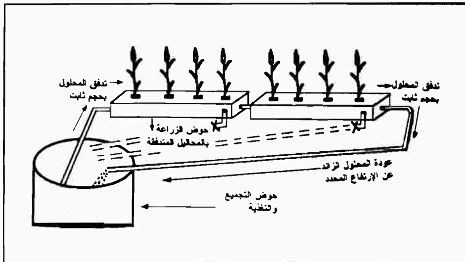
شكل (١٠ - ٢): أحواض الزراعة بالمحاليل المغذية المتدفقة ذات الحجم الثابت
