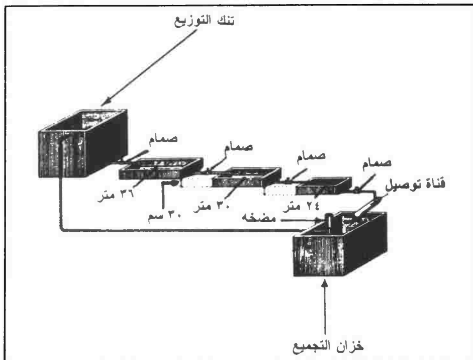
شكل (١٠ - ١٤): الرى بنظام الشرفات
