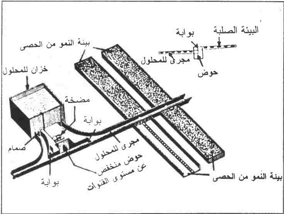
شكل (١٠-١٥): الري تحت السطحي بنظام القنوات
