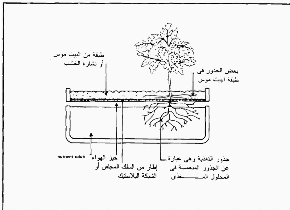
شكل (١٠ - ١): نموذج لزراعة محاليل مغذية ساكنة كما استخدمها Gericke
