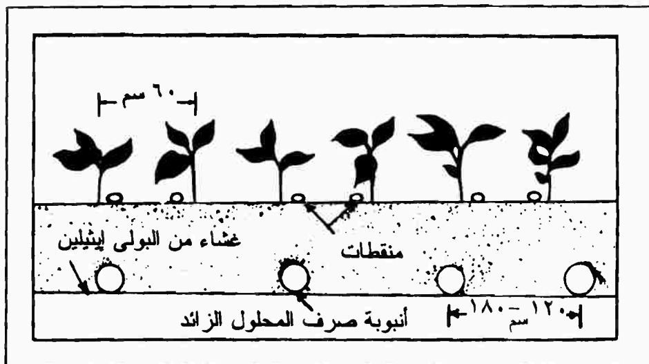
شكل (١٠-١٩) : قطاع عرضي لأرضية صوبة تم فرشها بالكامل ببينة الرمل
