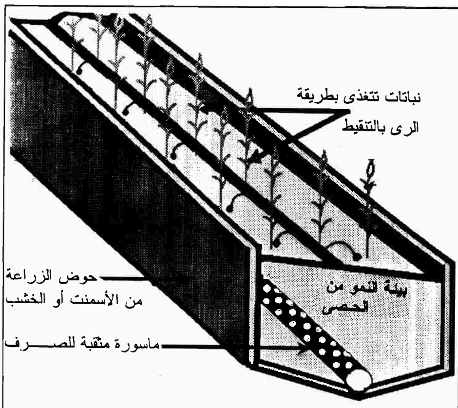
شكل (١٠-١٦): الرى بالتنقيط في مزارع الحصى
