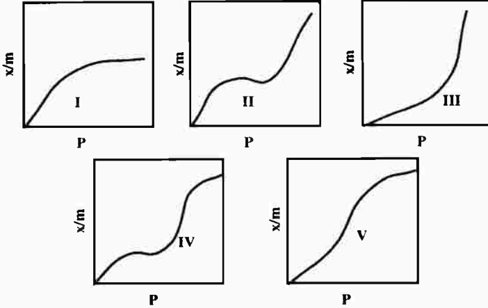
أنصاف أيزوثيرمات الامتزاز
