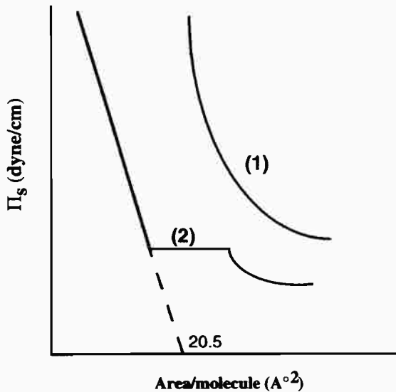
العلاقة بين ضغط السطح والمساحة لكل جزيء
