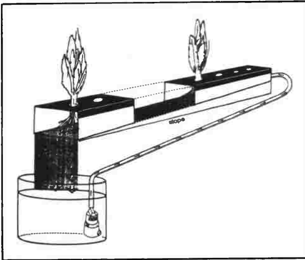
شكل (٥ - ١١) : الشكل العام لقناة الزراعة والتغذية بالأغشية المغذية
