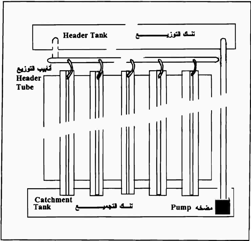
شكل (٥ - ٢٥): رسم تخطيطي لنظام الأغشية المغذية في مدينة السادات
