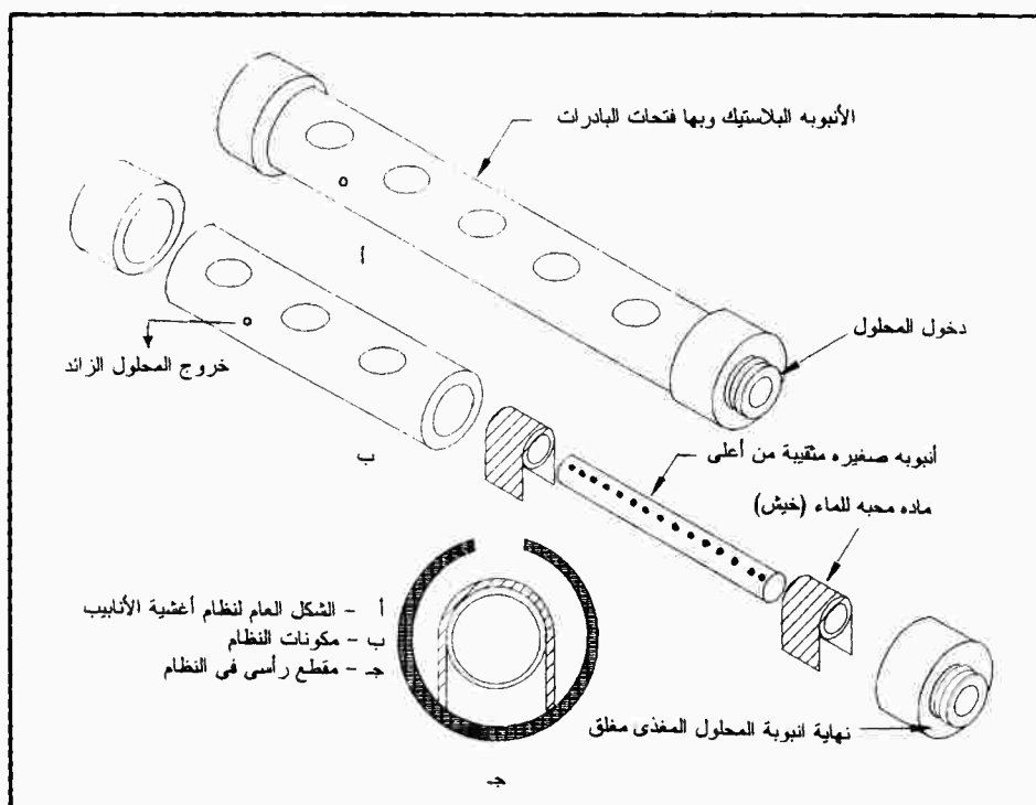
شكل (٥ - ٣١): طريقة أغشية الأنابيب واستخدام الخيش كمادة ماصة فى المحلول المغذى
