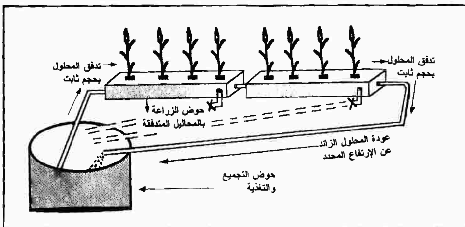
شكل (٧-٥) : أحواض الزراعة بالمحاليل المغذية المتدفقة ذات الحجم الثابت
