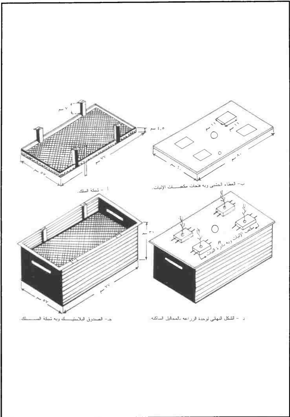
(شكل ٥-٢) : رسم تخطيطي لمكونات احدى وحدات الزراعة فى المحاصيل المغذية الساكنة فى الصوبة
