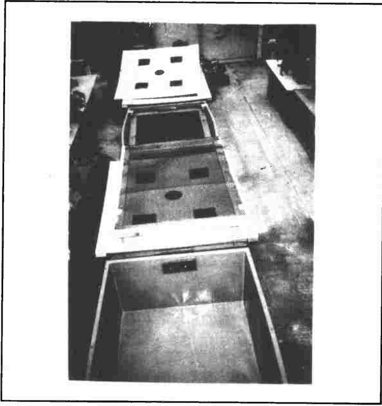
شكل (٥ - ٣) : أحواض الزراعة فى المحاليل الساكنة وكيفية إعدادها للزراعة
