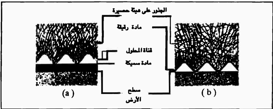
شكل (٥ - ١٦): تأثير سمك غشاء البوليثلين على درجة التصاقه بقاعدة حصيرة الجذور فى قنوات الأغشية المغذية
