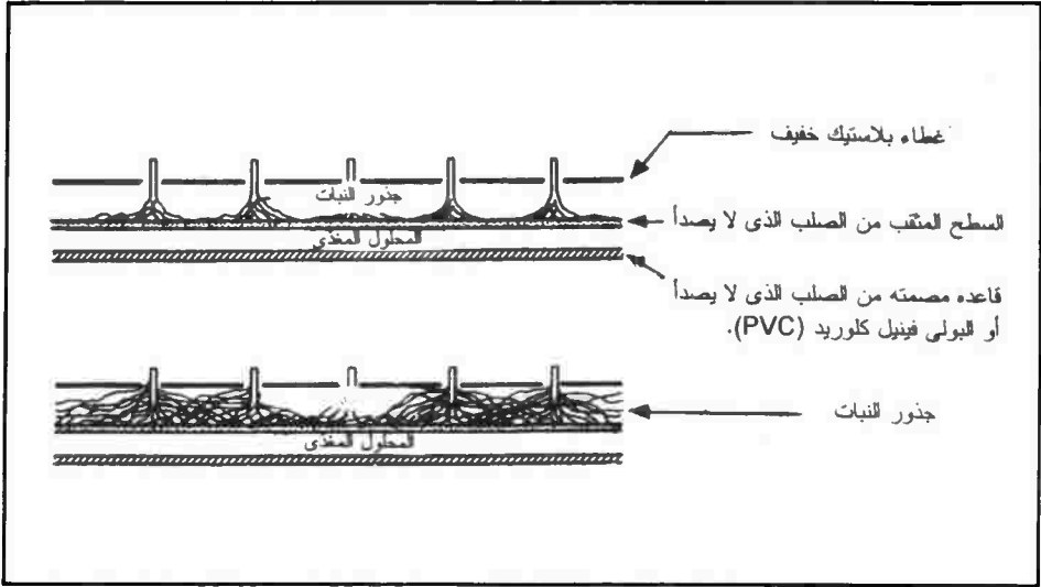
شكل (٥ - ٣٢): رسم تخطيطي للنظام الزراعي في الأغشية الماسمية
