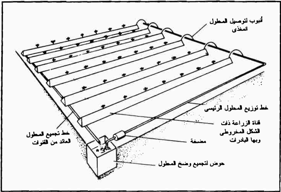
شكل (٥ - ١٢): التصميم العام لزراعة الأغشية للغذية NFT
