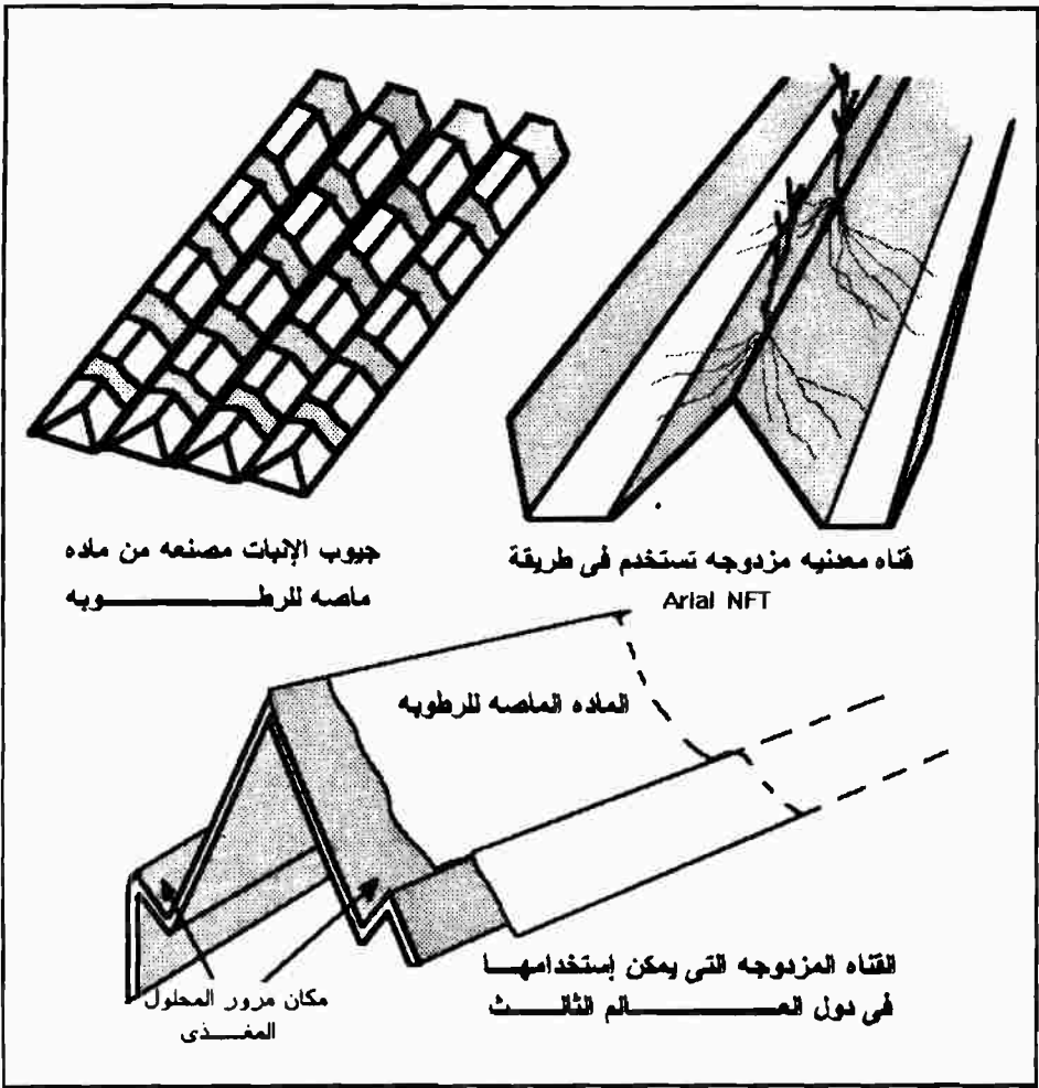
شكل (٥ - ٢٦): تحويل آخر لقنوات الأغشية المغذية ليساعد على الاستخدام فى المناطق الحارة
