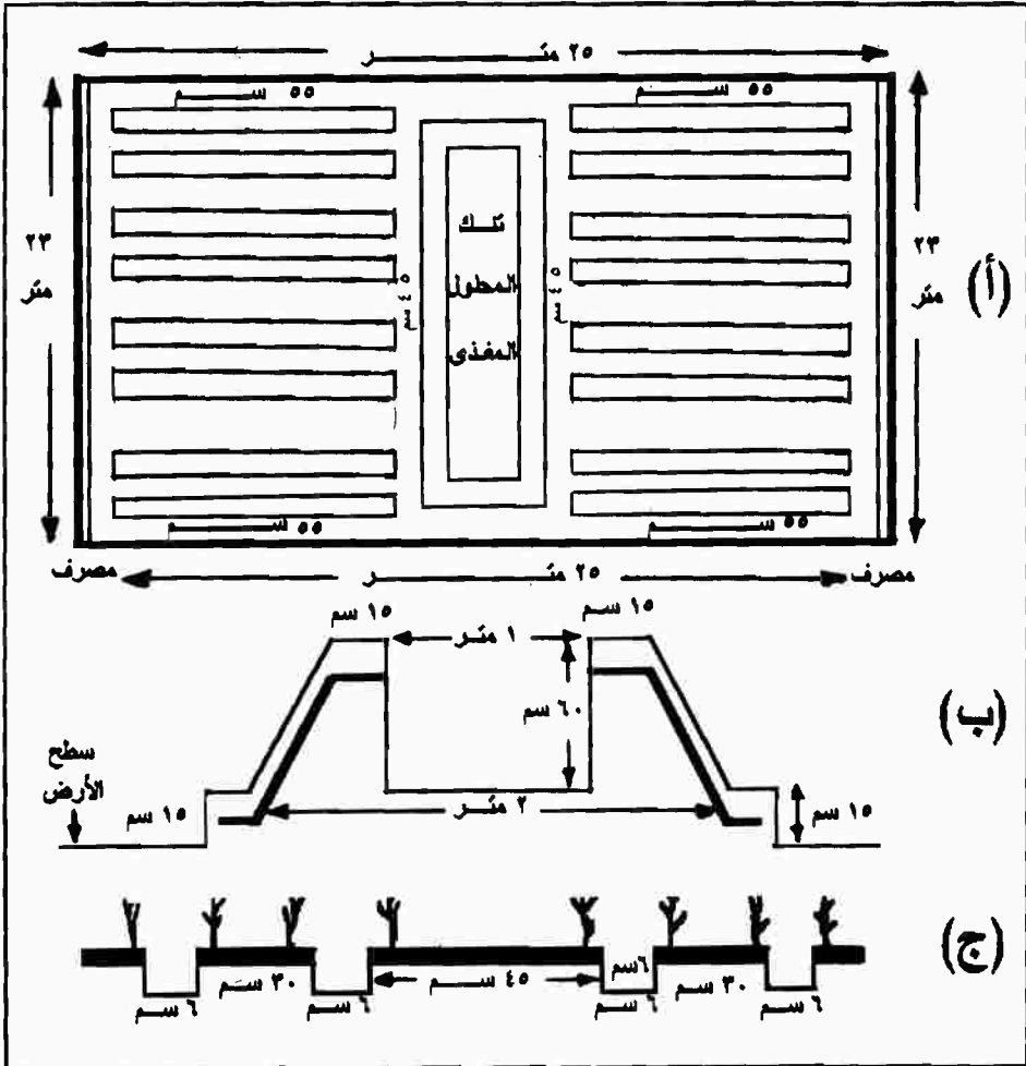
شكل (٥ - ٢٧): رسم تخطيطي للطريقة الهندية ونظام الأغشية المغذية
