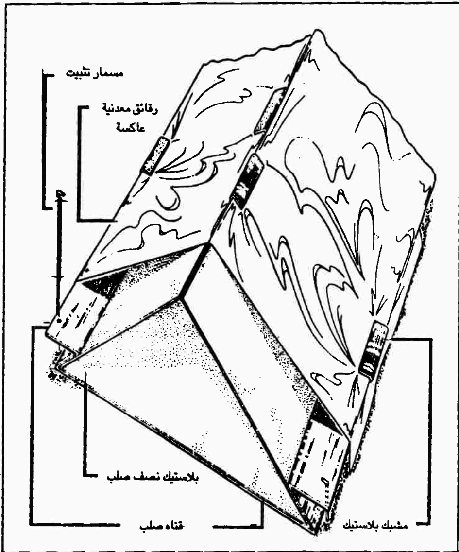
شكل (٥ - ١٣) : القناة القياسية في نظام الأغشية المغذية
