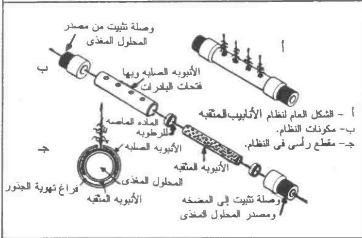
شكل (٥ - ٣٠): طريقة الأنبوب المشقبة ونمو نباتات القمح بها حتى عمر ثلاثة أشهر ونصف
