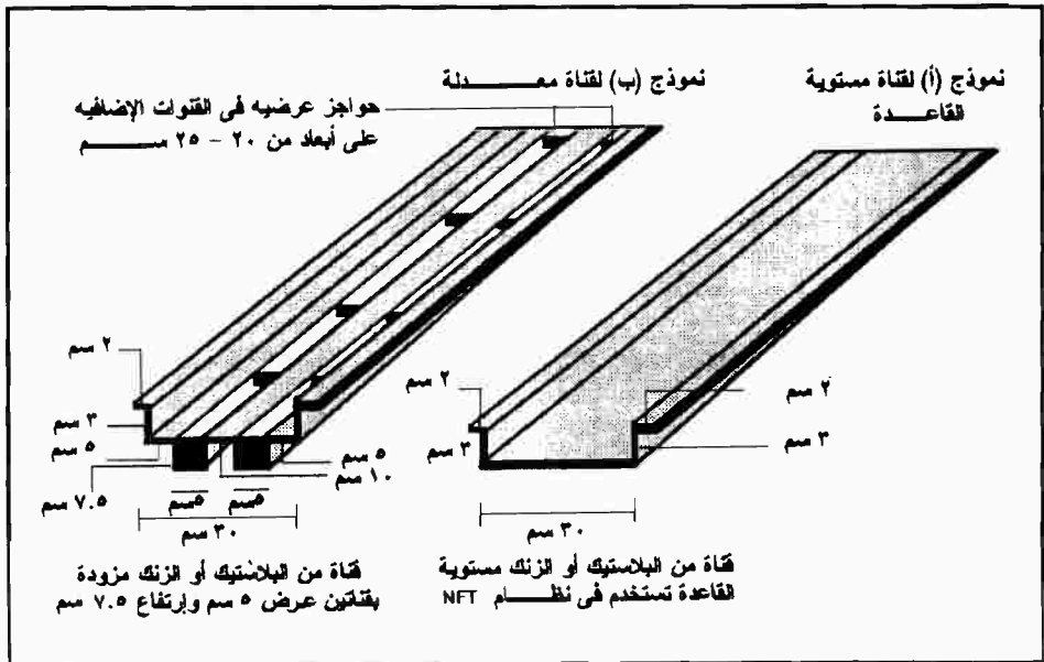
شكل (٥ - ٢٤): تحويل قناة الأغشية المغذية لتقليل خطر انقطاع التيار الكهربائي
