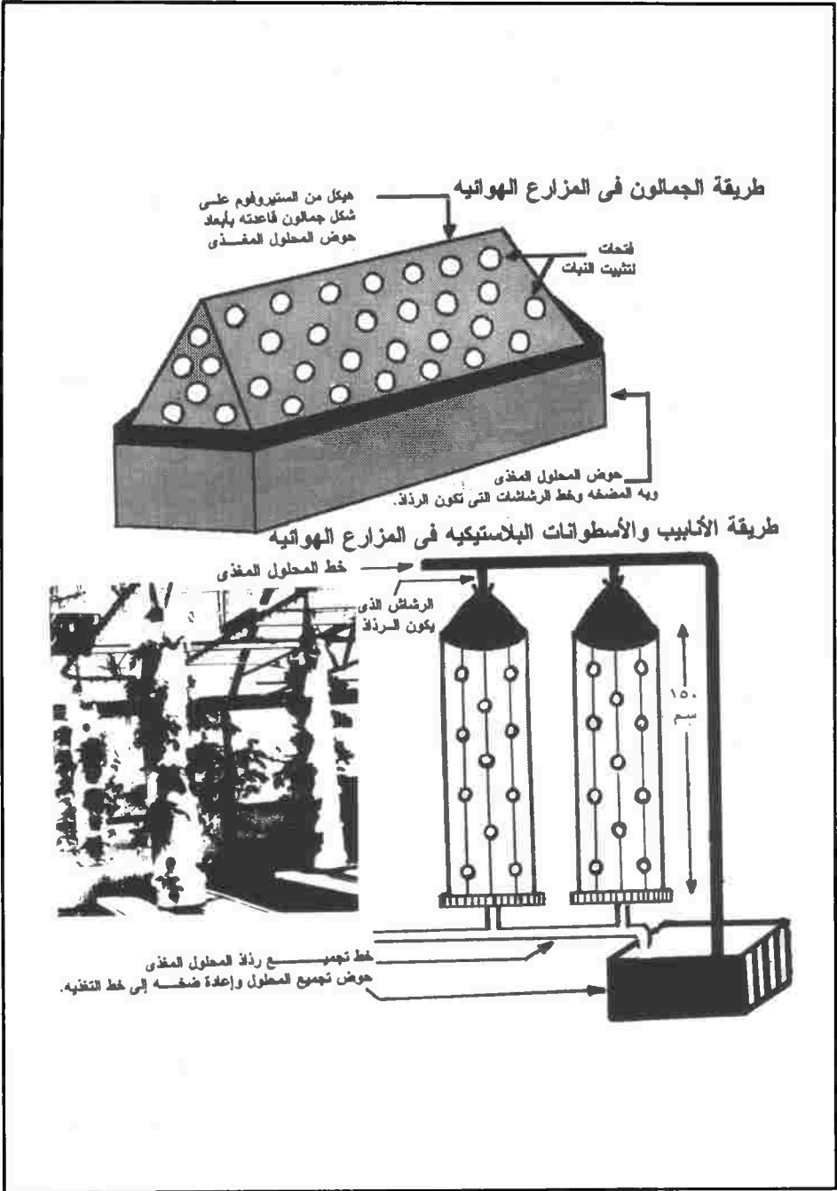
شكل (٥ - ٢٨): المزارع الهوائية بطريقة الجمالون (لأعلى) والأسطوانات الرأسية (لأسفل)
