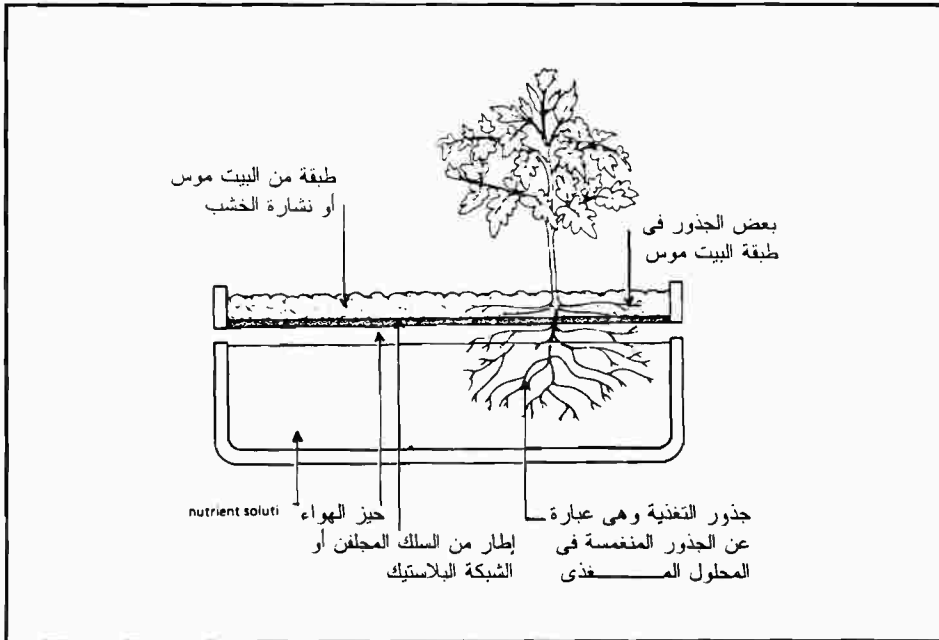
(شكل ١-٥) : نموذج لزراعة محاليل مغذية كما استخدمها Gericke
