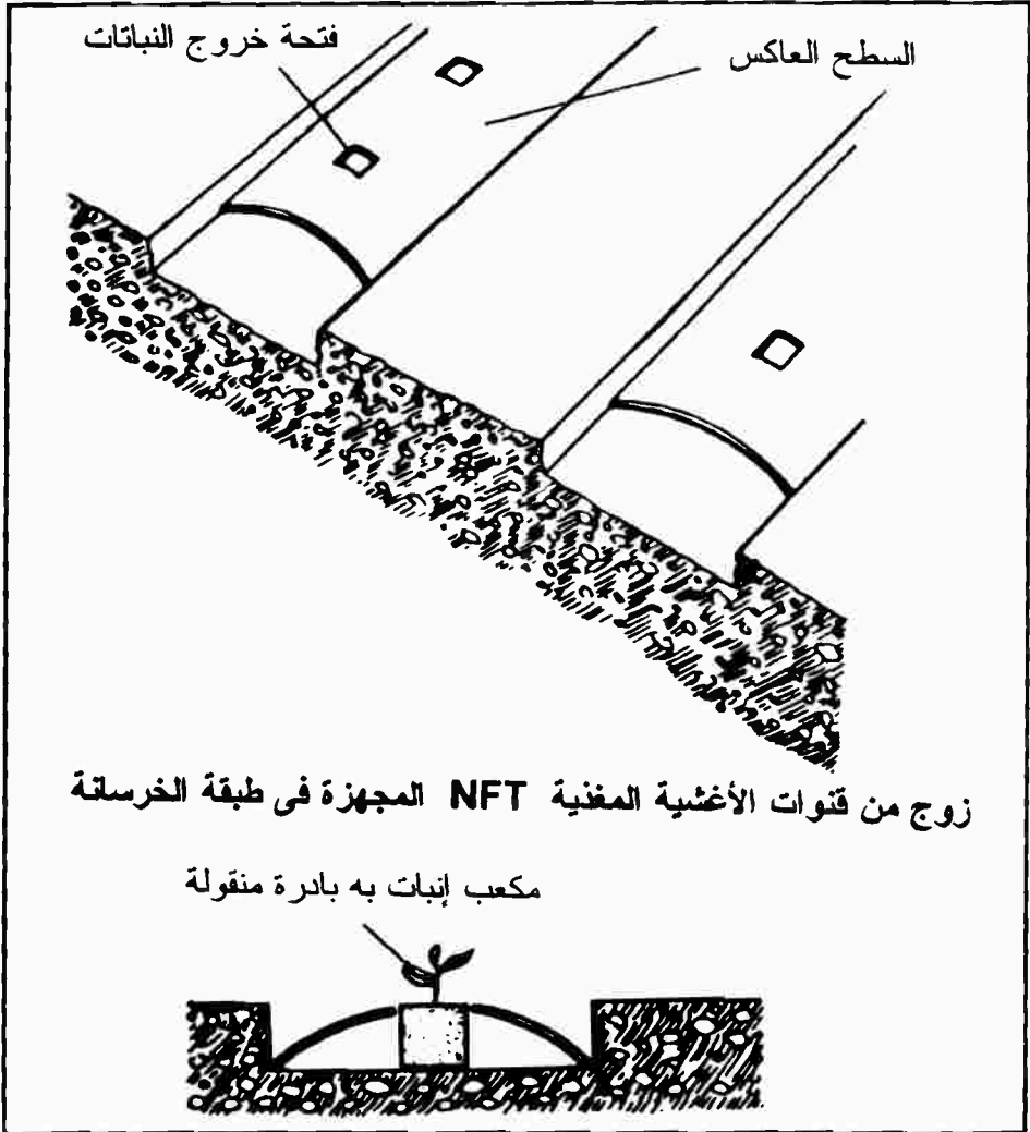
شكل (١٤-٥): زوج من قنوات السطح المجهز المغطاة بسطح معدني عاكس
