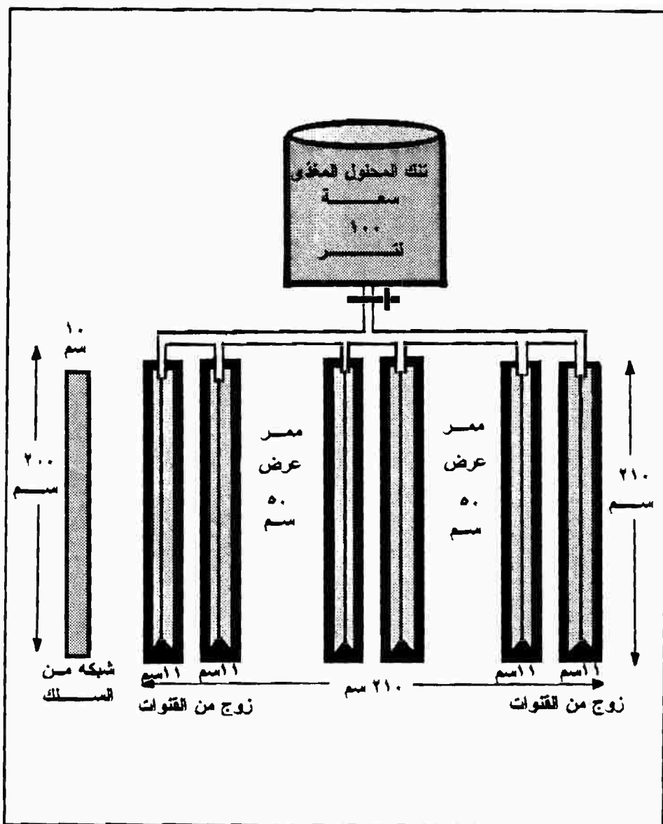
شكل (٥-٦) : رسم تخطيطي لمزرعة محاليل ساكنة في الحقل المفتوح
