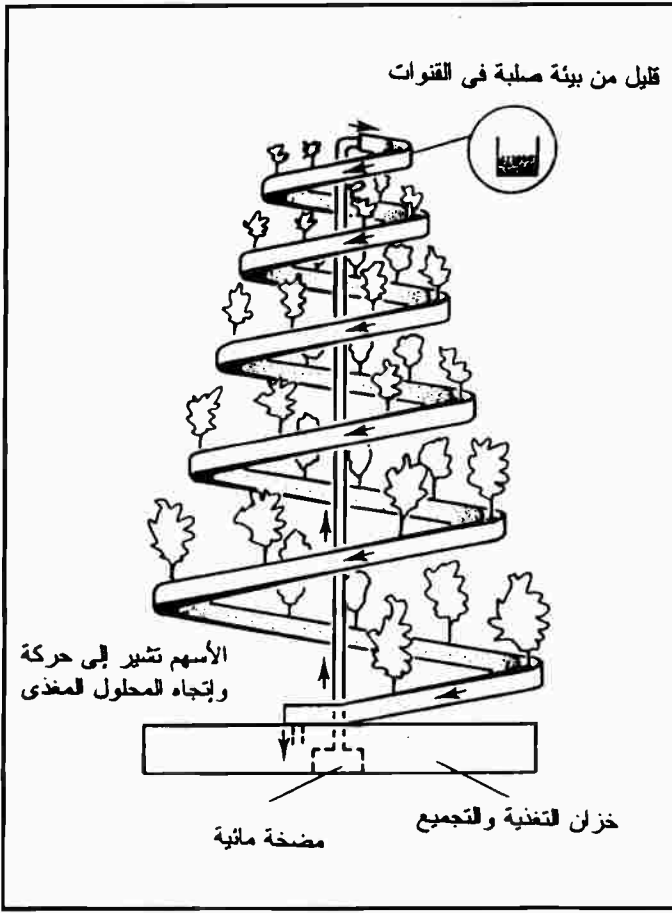
شكل (٨-٢١): الحديقة الحلزونية ونظام الزراعة في الأغشية المغذية
