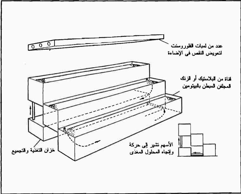
شكل (٨-١٩) وحدات زراعة بنظام الأغشية المغذية متعددة الأدوار
