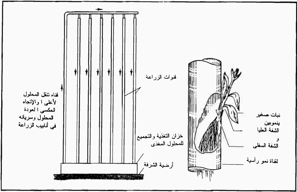
شكل (٨-٢٠) : وحدات رأسية من الأنابيب تستخدم للزراعة بنظام الأغشية المغذية
