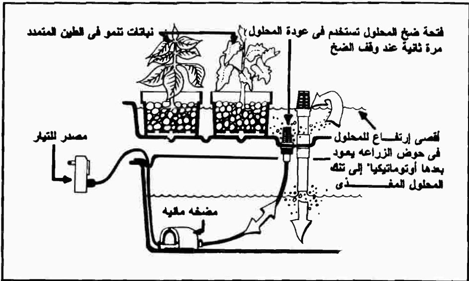
شكل (٨-١٠): ميكانيكية الري والتغذية تحت السطحي لوحدة الزراعة الأفقية في أصص
