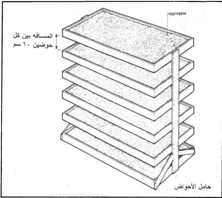
شكل (٦-٨) : طريقة الزراعة فى أحواض البيئات الصلبة الرأسية فى المنزل
