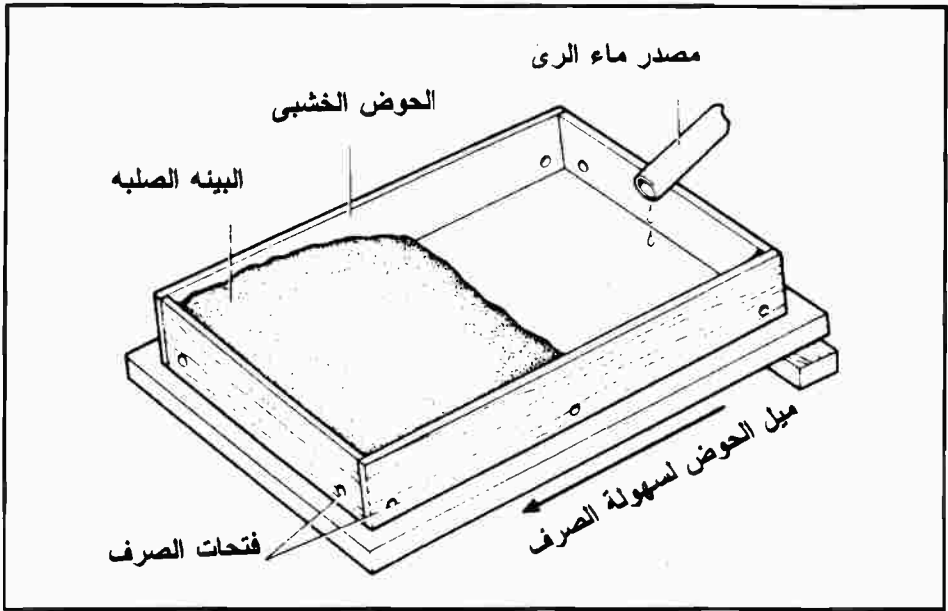
شكل (٨-٥): يوضح كيفية وضع بيئة النمو في الأحواض الخشبية وطريقة الري السطحي
