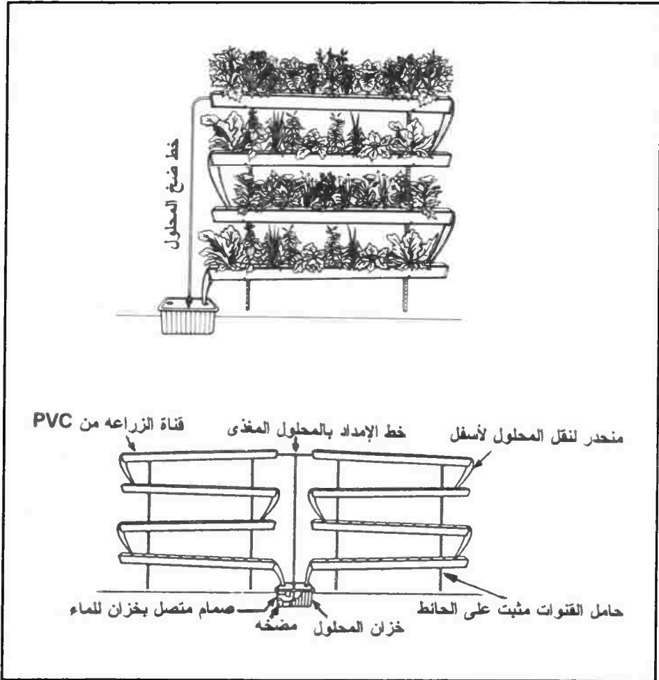
شكل (٨-١٧): وحدات رأسية لنظام الزراعة في الأغشية المغذية تصلح للتثبيت على الحوائط وفي الأركان
