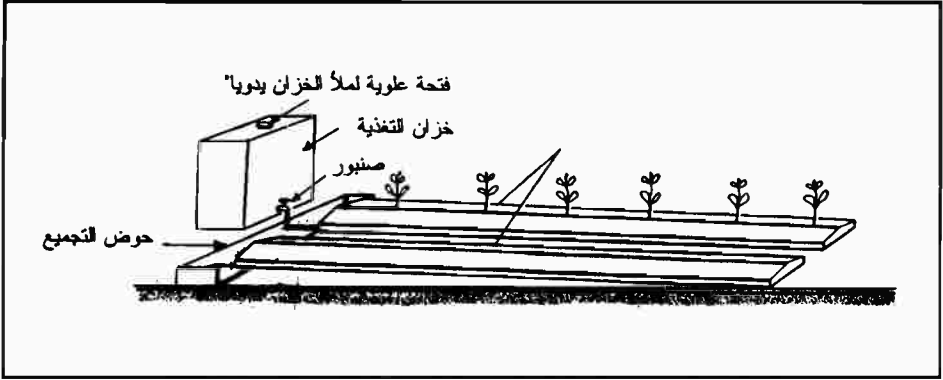
شكل (٨-١٥) : وحدة زراعة بنظام الأغشية المغذية تعمل بطريقة يدوية
