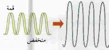
تداخل إيجابي يكون ضوءاً أعمق
