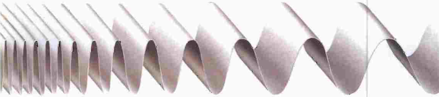
اشعة جاما
