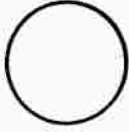
جزيء الحديد Fe = ذرة حديد
