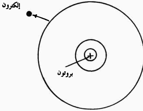
شكل (٢ - ٤) (أ) أيون هيدروجين موجب (بروتون) أي ذرة هيدروجين فقدت إلكترون
