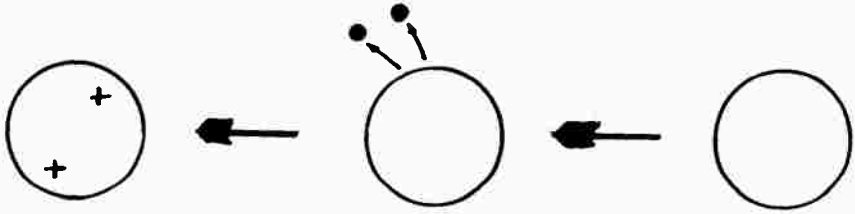
عند فقدان عدد ٢ إلكترون تصبح أيون ثنائي موجب
