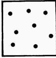
الذرات في الحديد
