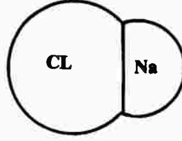
جزء من كلوريد الصوديوم عبارة
