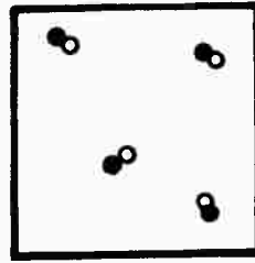
جزيئات كبريتيد الحديد
