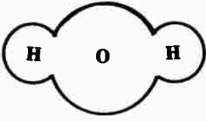
جزء ماء عبارة عن
