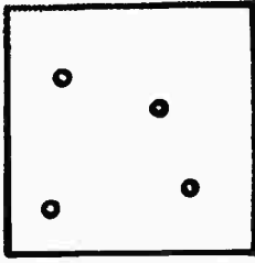
الذرات في البوتاسيوم
