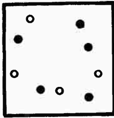
الذرات في خليط من الحديد والبوتاسيوم
