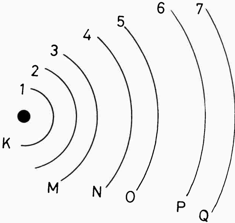
شكل (٢ - ٣) مدارات الإلكترونات حول النواة
