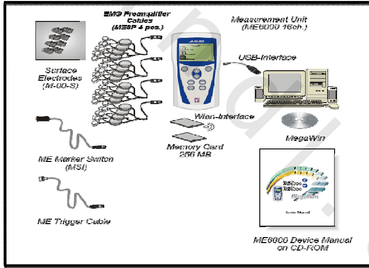
شكل (٨) مكونات جهاز رسام النشاط الكهربى للعضلات اللاسلكى (EMG)
